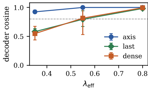
GPT-2 SAE cosine
