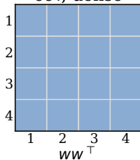
cov, dense
