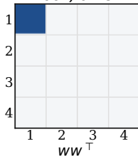
cov, axis
