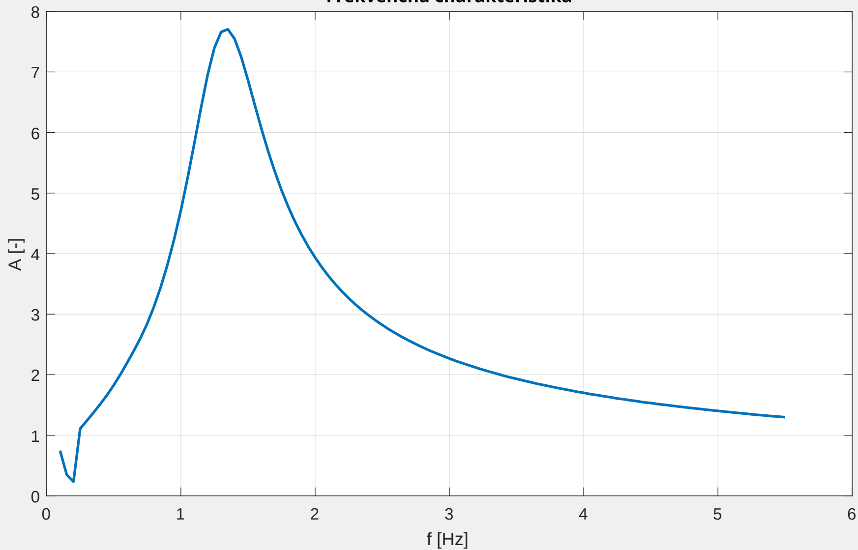
Frekvenčná charakteristika
