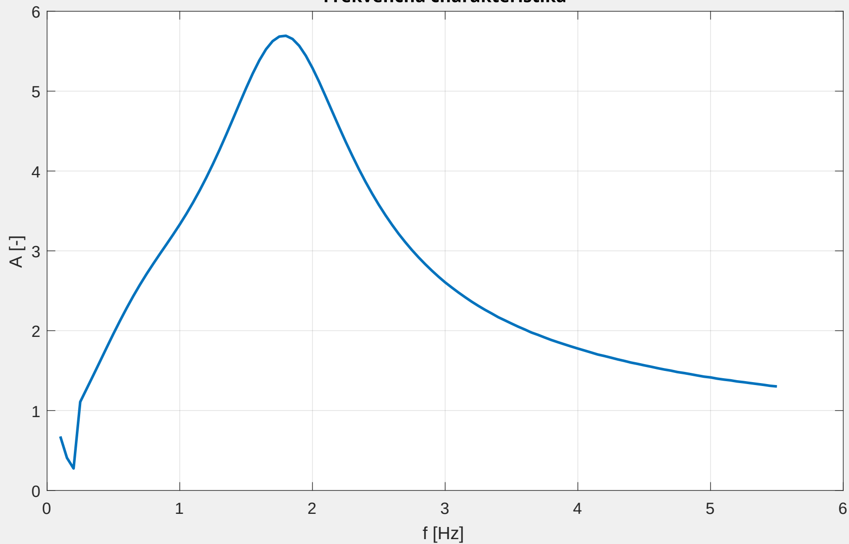
Frekvenčná charakteristika
