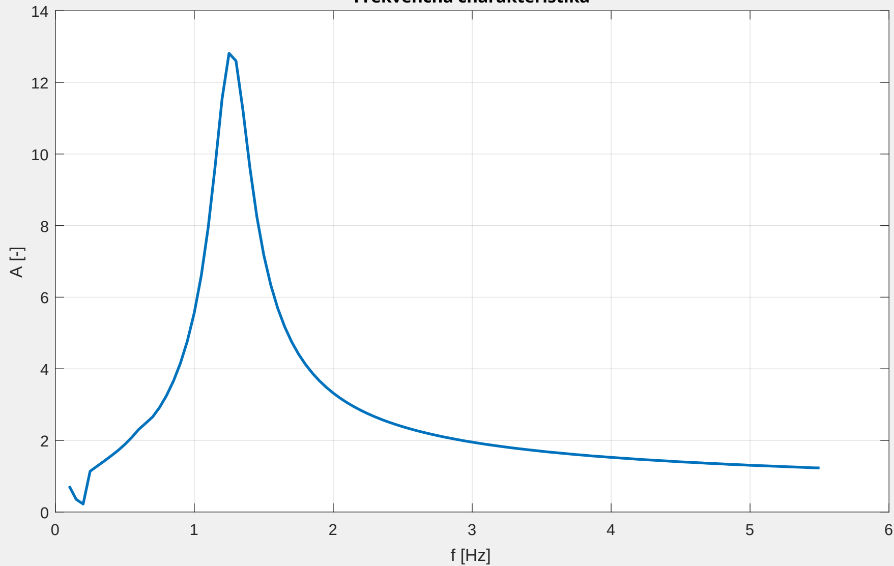
Frekvenčná charakteristika
