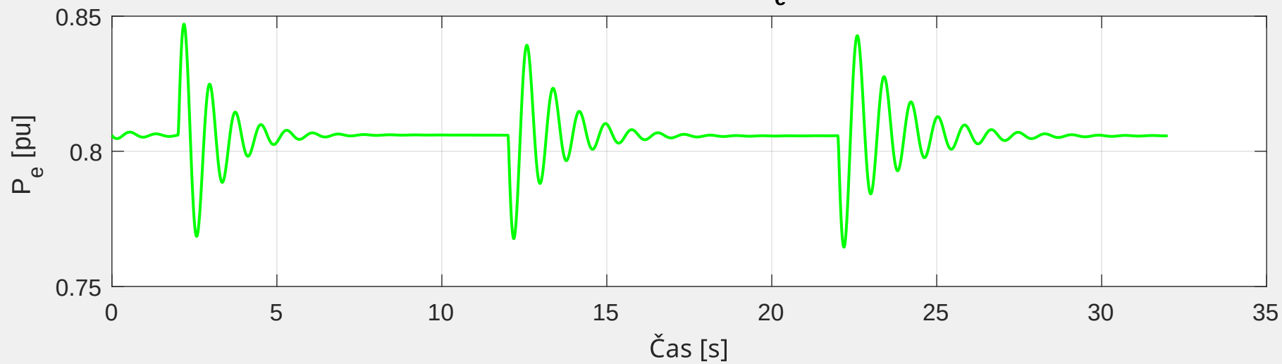
Činný výkon ( P_e )
