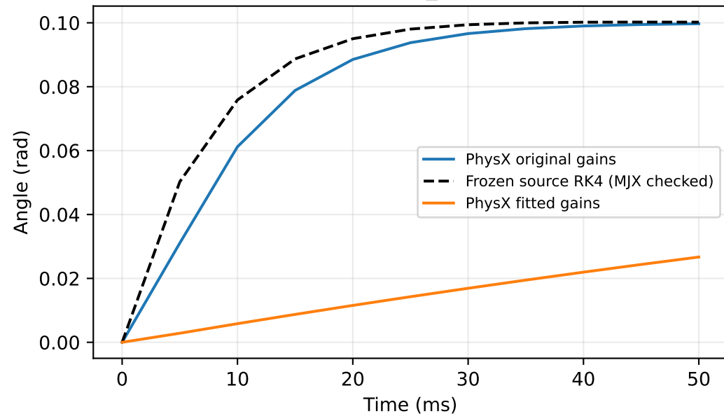
steering_joint
