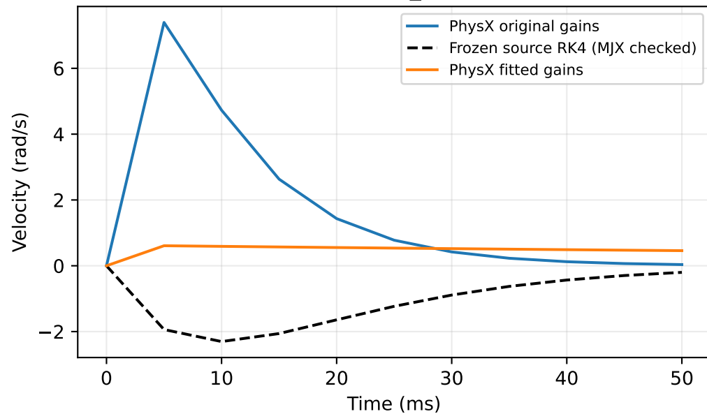
steering_joint
