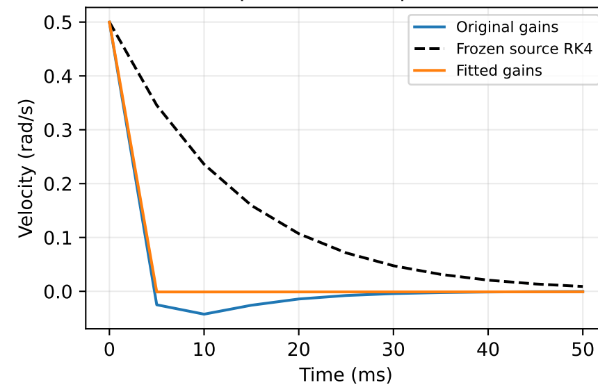
steering_joint input=0, initial qd=0.5
