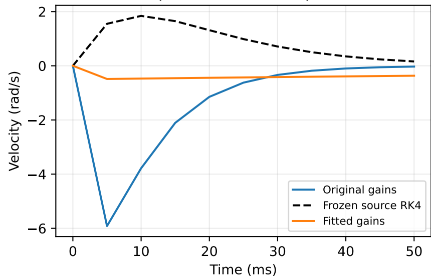
steering_joint input=-0.08, initial qd=0
