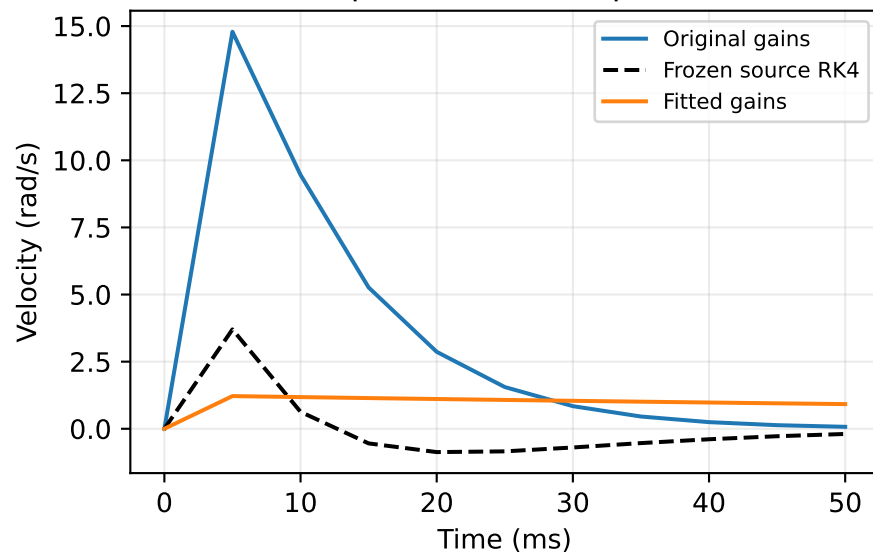
steering_joint input=0.2, initial qd=0
