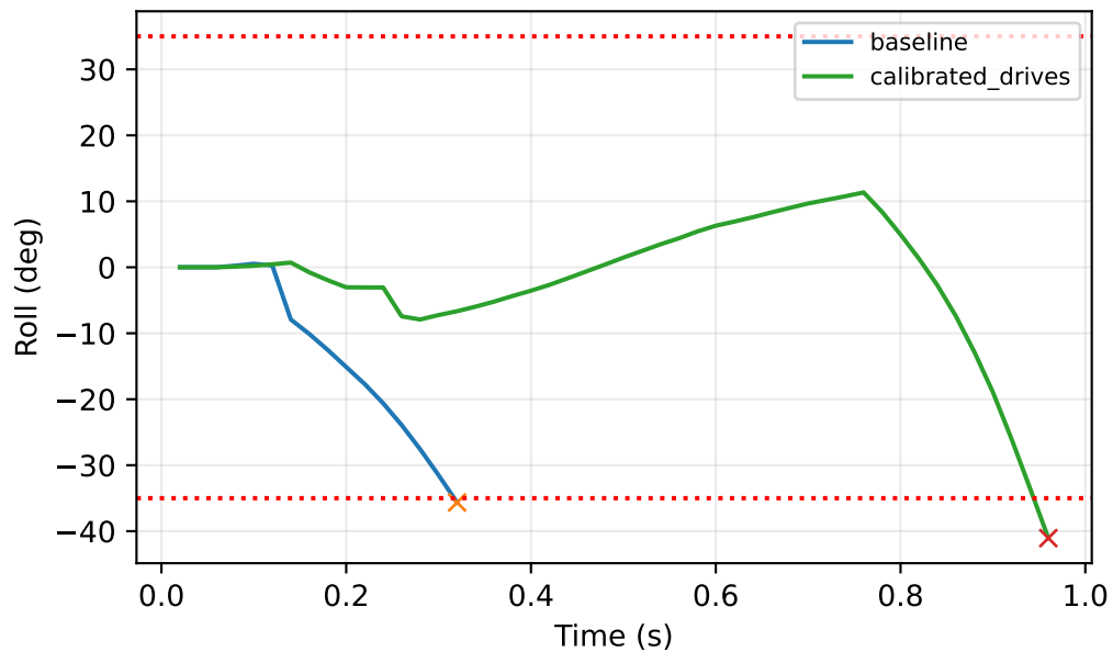
Actual roll-limit failures
