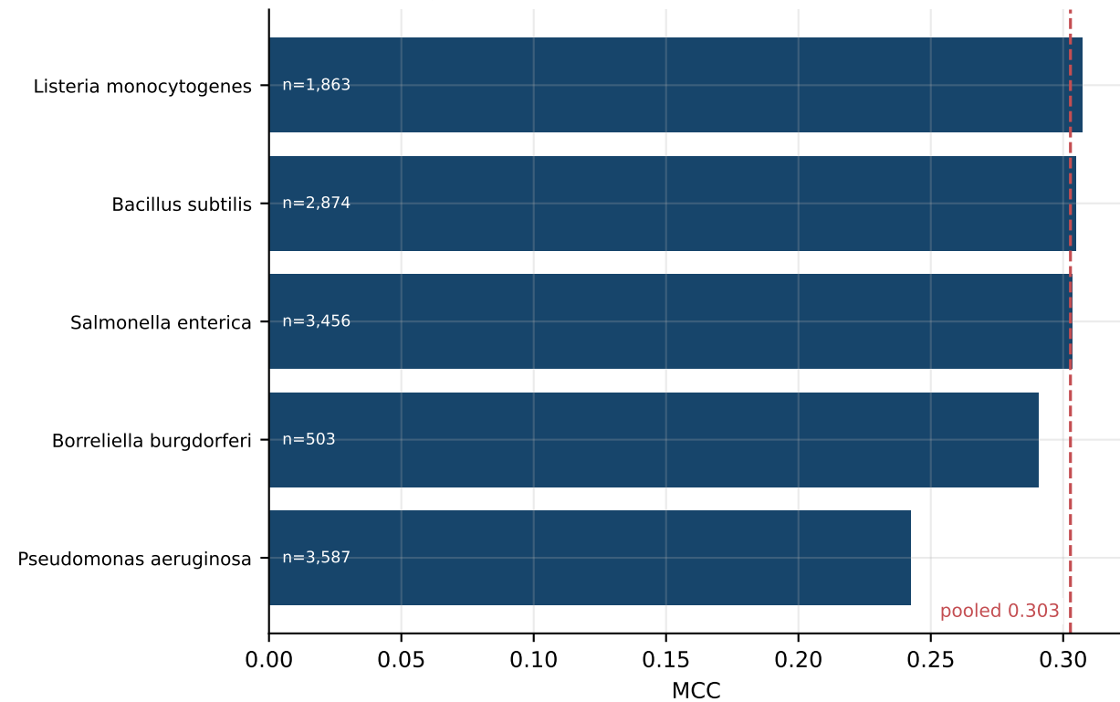
Per held-out genome
