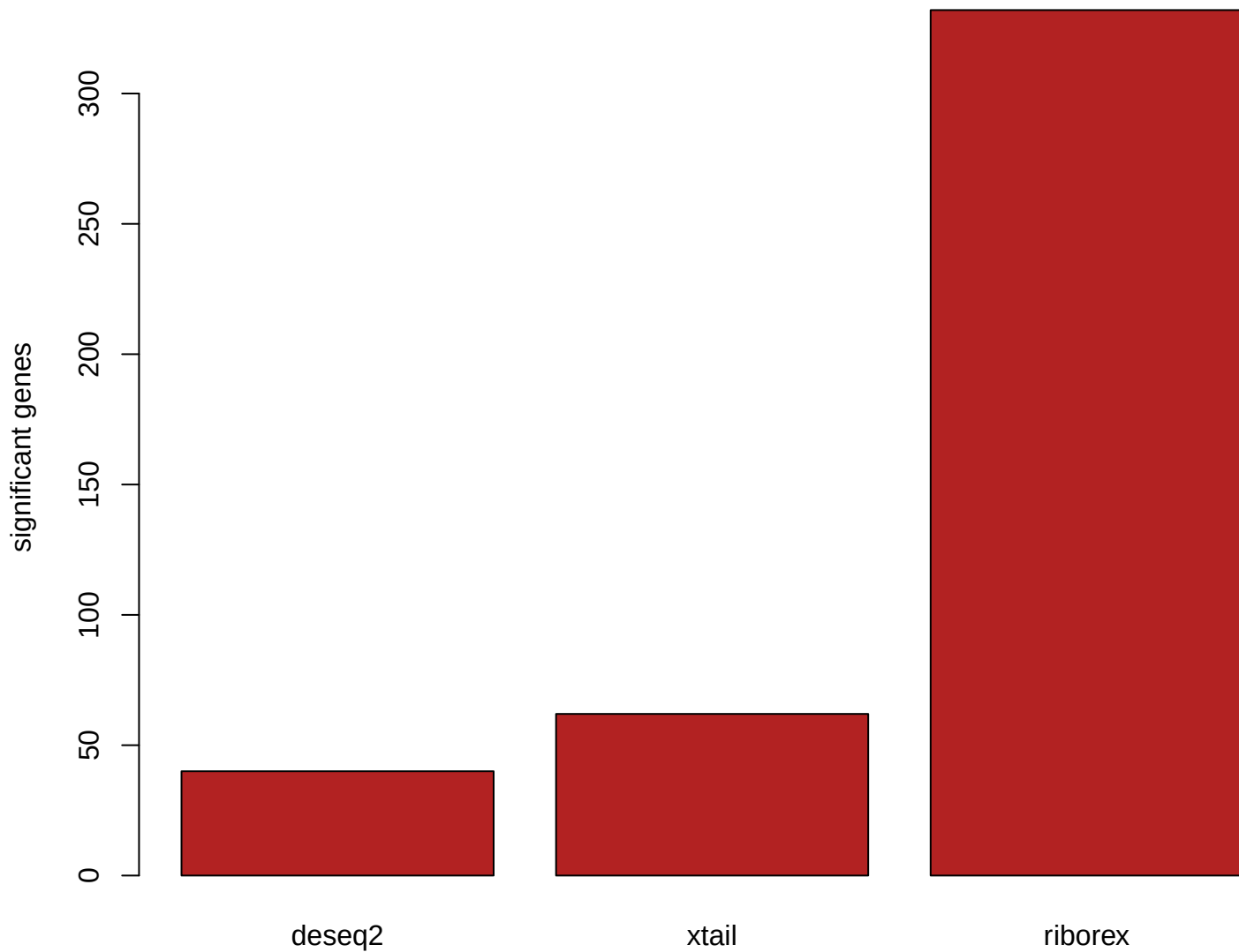
TE hits per method (padj < 0.05)
