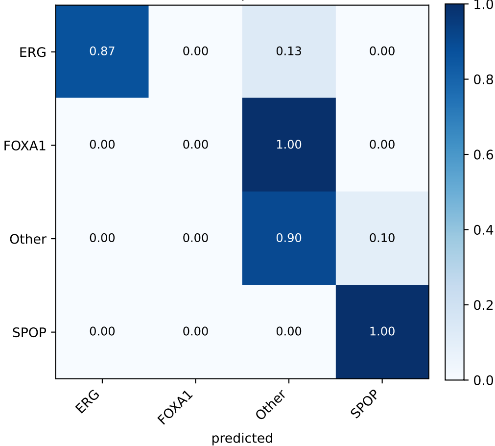
PRAD mixup (seed 46)
