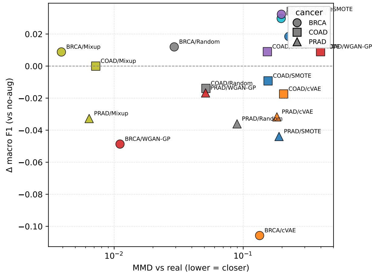
Distribution match (MMD) vs downstream \Delta F1
