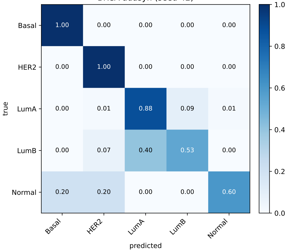
BRCA adasyn (seed 42)
