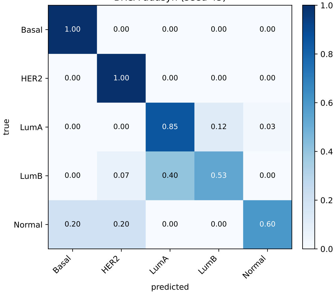
BRCA adasyn (seed 43)
