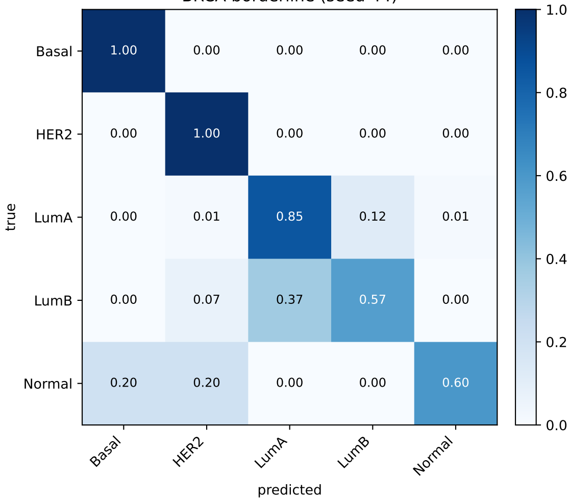
BRCA borderline (seed 44)
