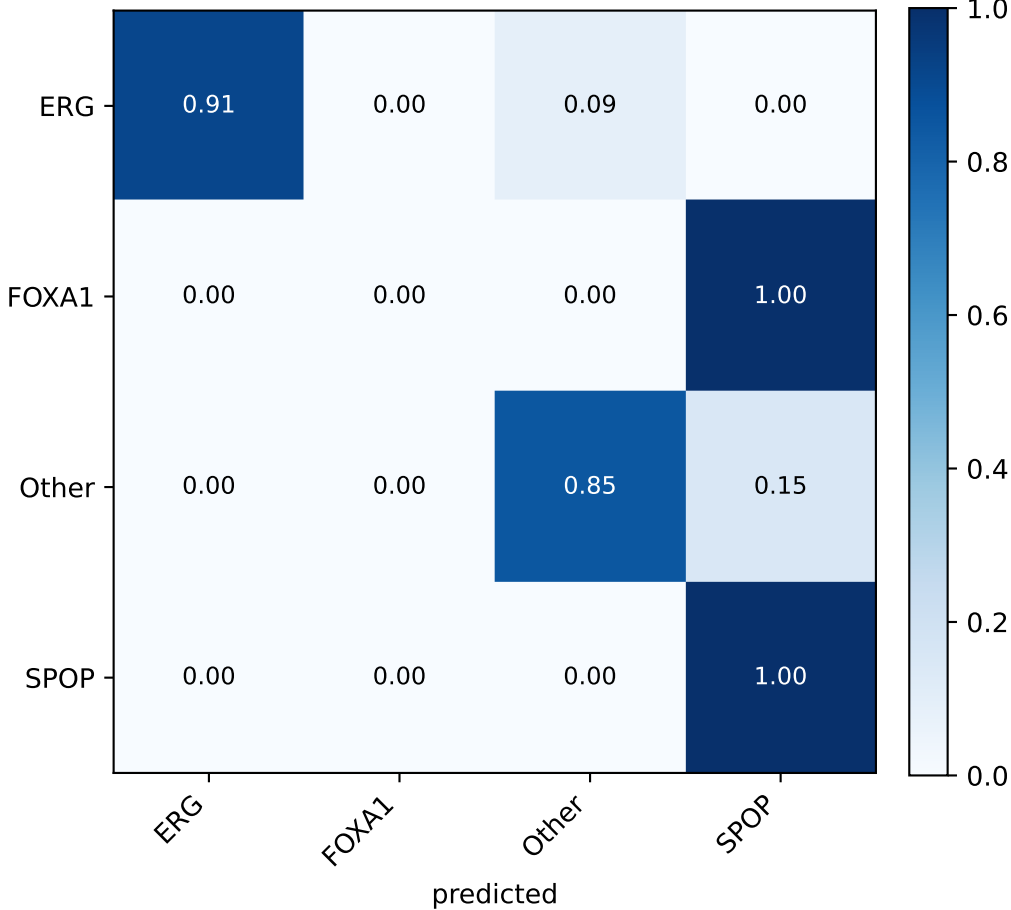
PRAD borderline (seed 45)
