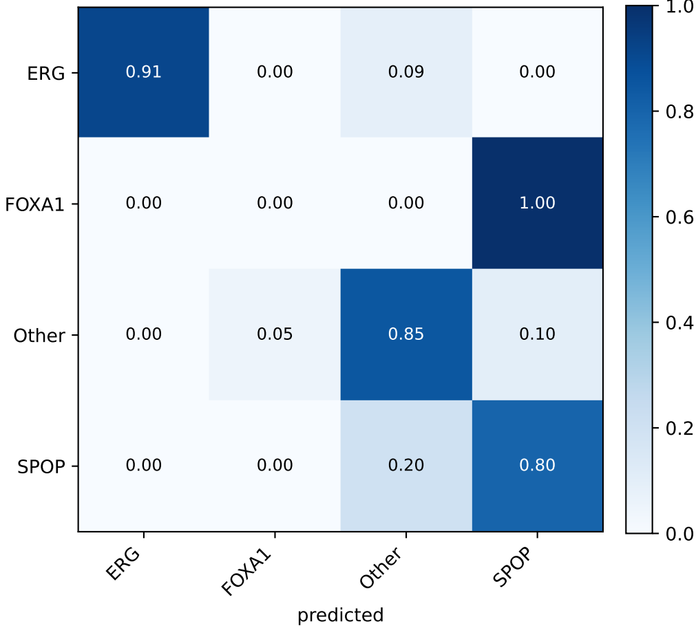
PRAD random (seed 45)
