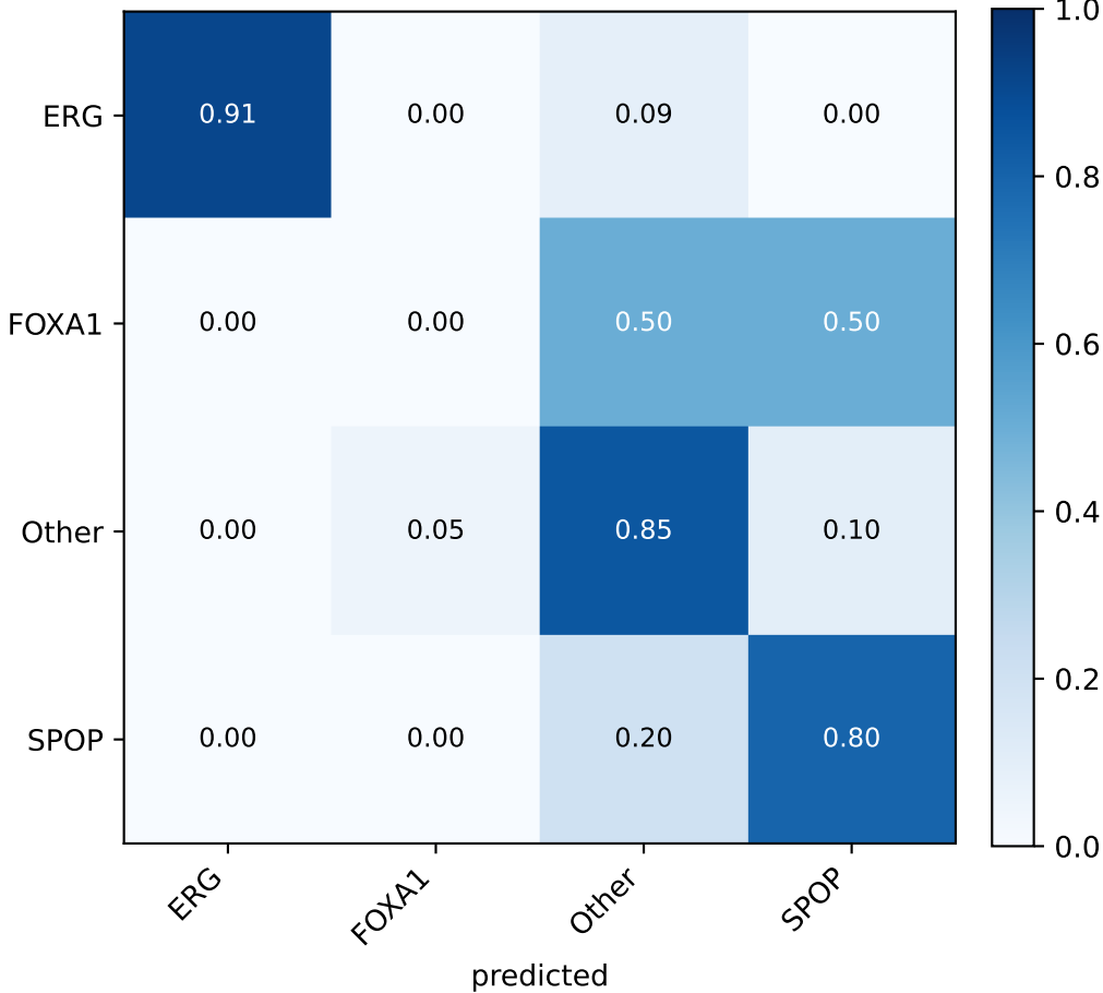
PRAD smote (seed 45)
