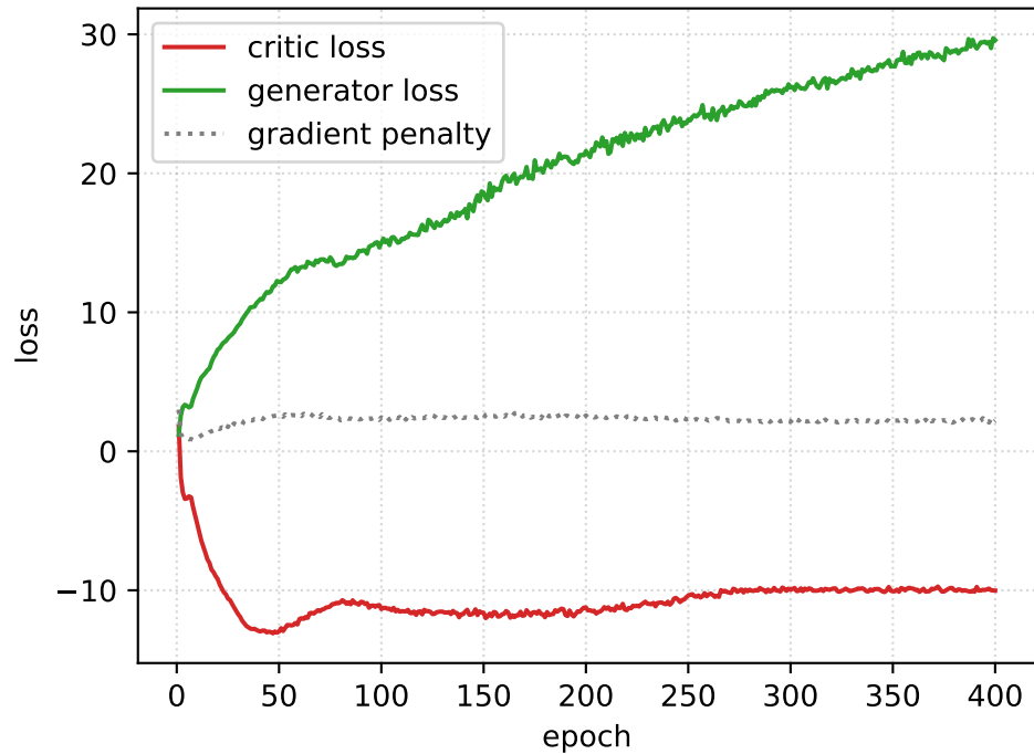
BRCA WGAN-GP — D / G / GP
