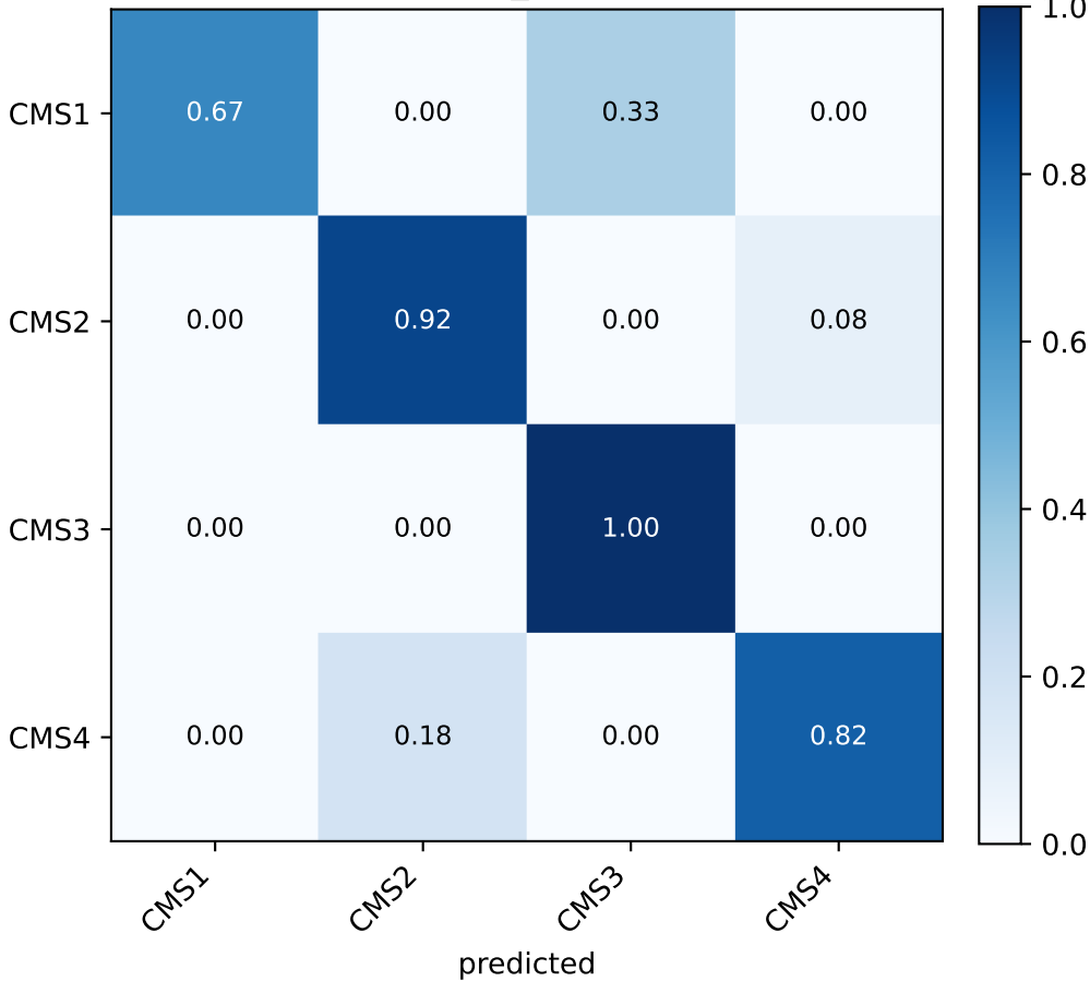
COAD wgan_gp (seed 43)
