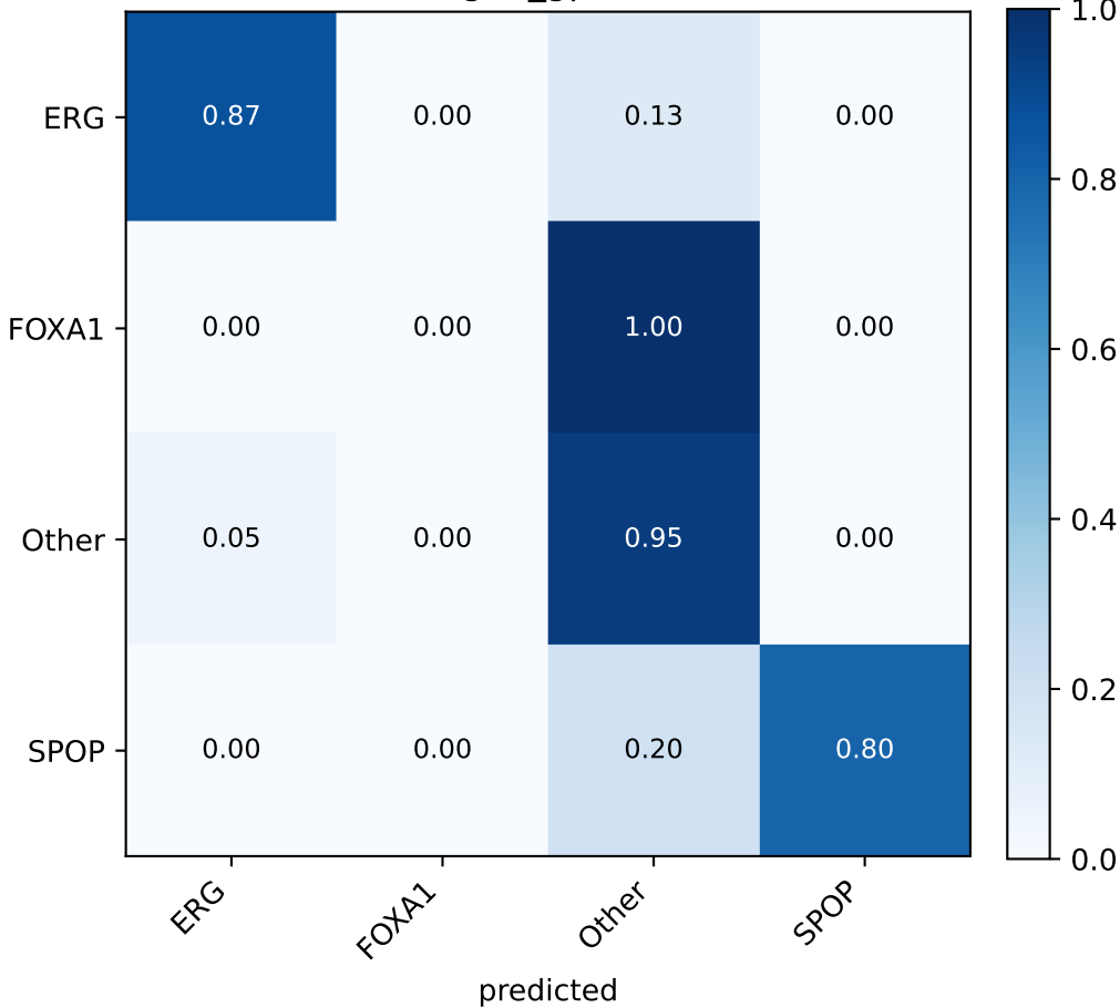
PRAD wgan_gp (seed 46)
