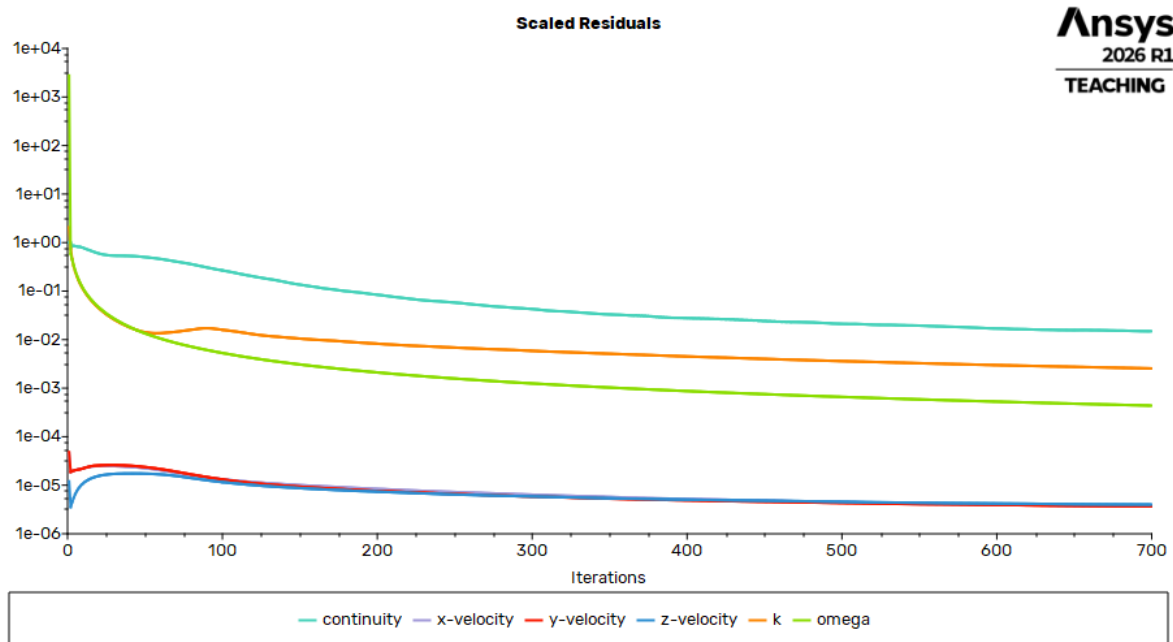
Rysunek 6.3: Przebieg residuów dla V_\infty = 10 m/s, n = 3000 RPM.
