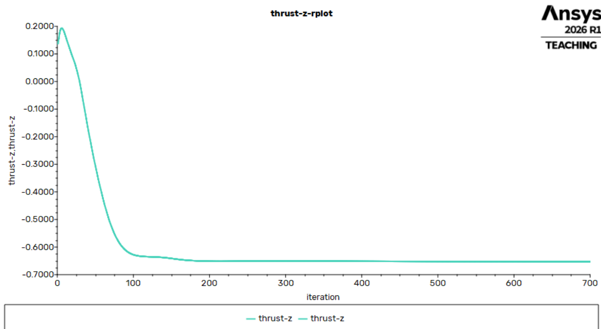
Rysunek 6.4: Przebieg ciągu (Thrust) dla V_\infty = 10 m/s, n = 3000 RPM.
