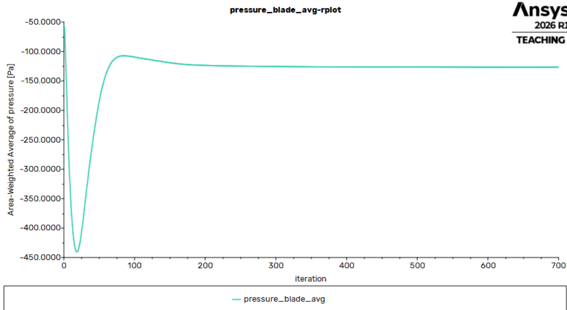
Rysunek 6.5: Średnie ciśnienie statyczne na łopatkę dla V_\infty = 10 m/s.
