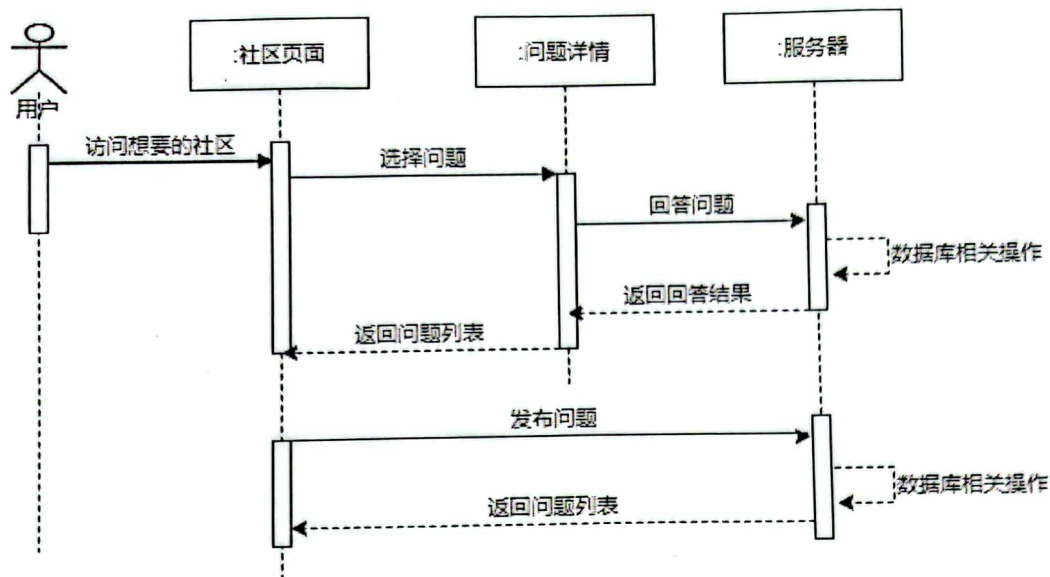
图 2.2 问答时序图
