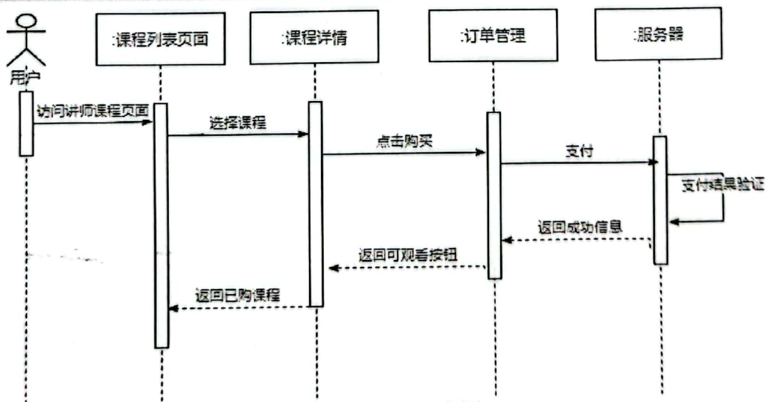
图 2.1 购课时序图
