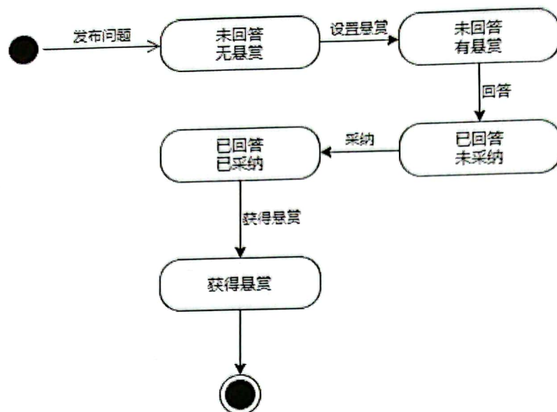
图 5.1 问答状态图
