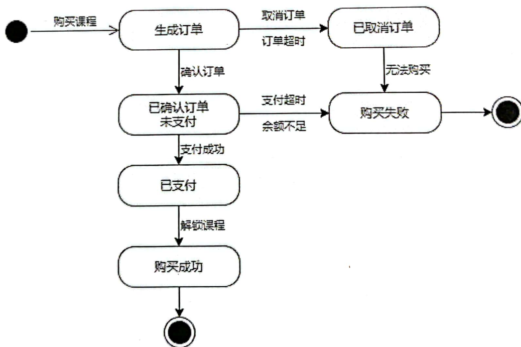
图 5.1 购课状态图
