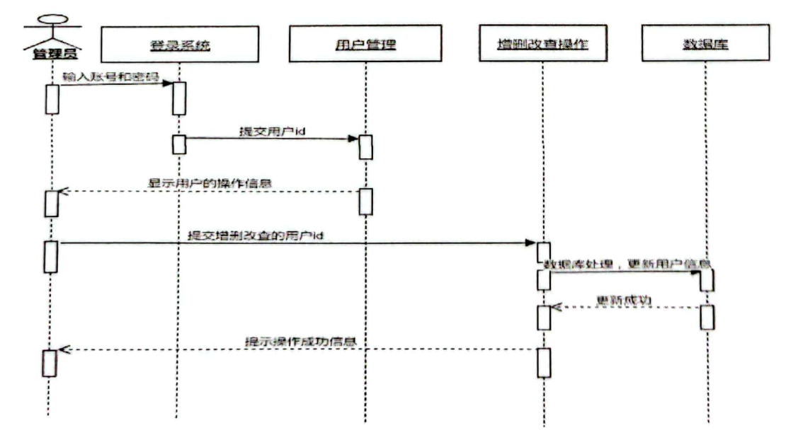
图 10 管理用户时序图
