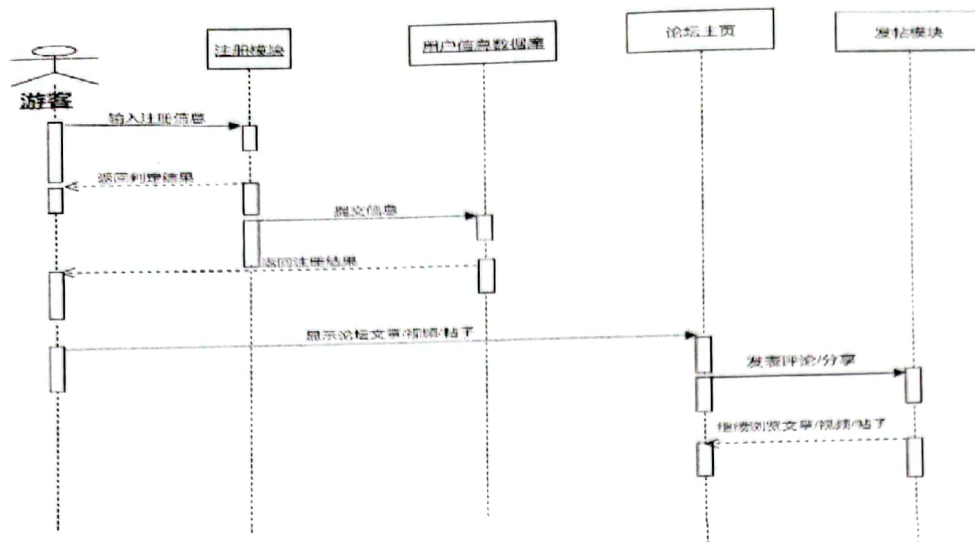
图 8 游客注册/登录时序图
