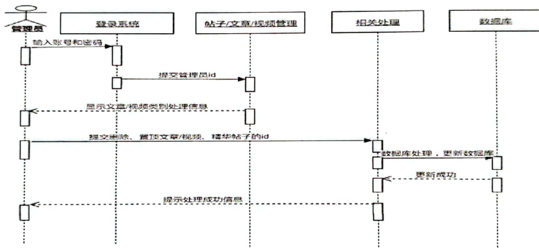
图 12 管理帖子/文章/视频的时序图
