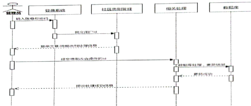
图 11 管理分类模块时序图
