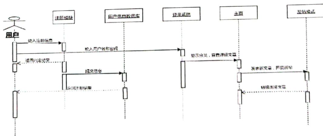
图 9 用户注册/登录、发帖回帖时序图
