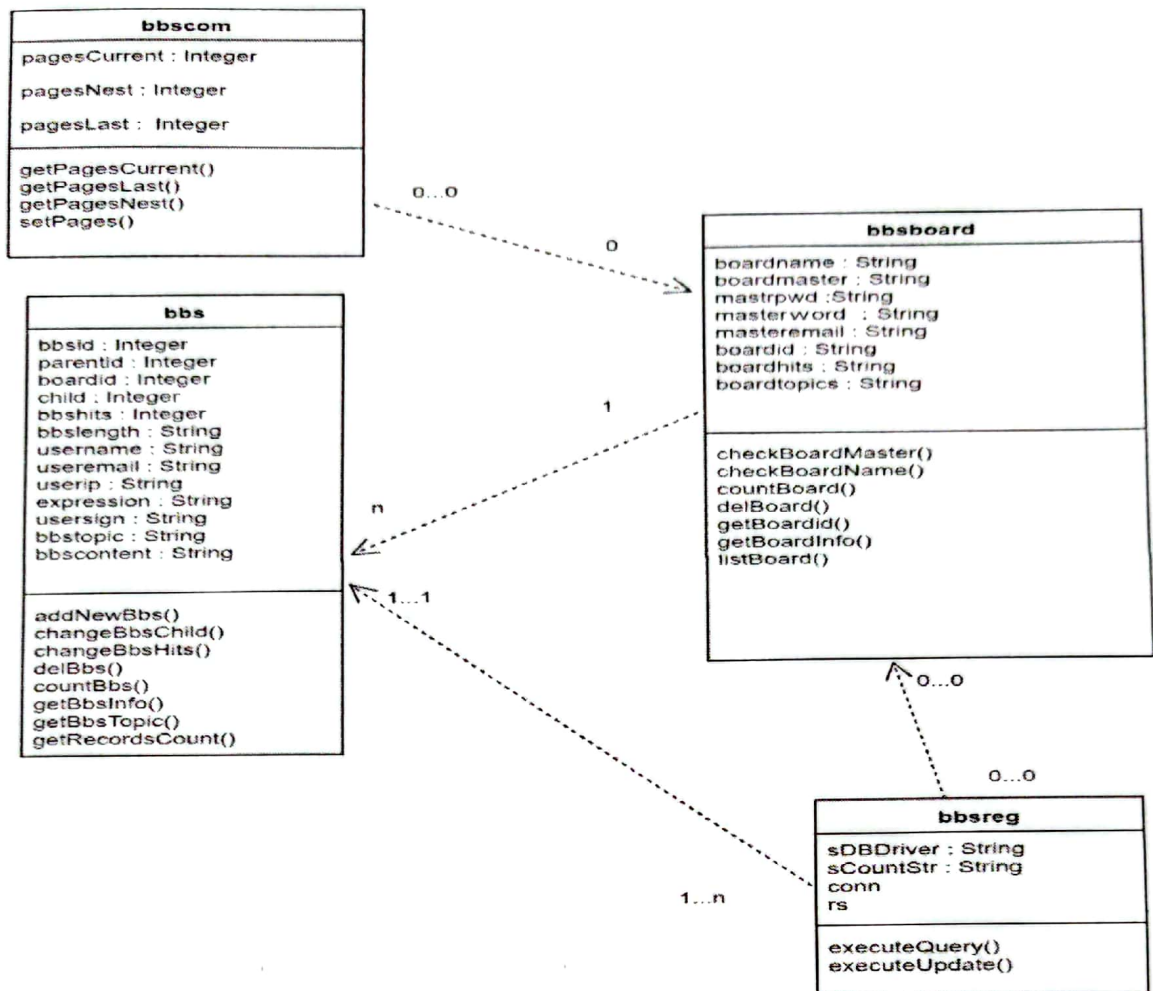
图 7 系统类图
