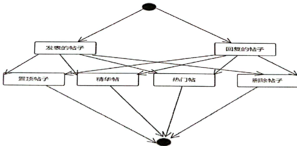
图 14 内容状态图
