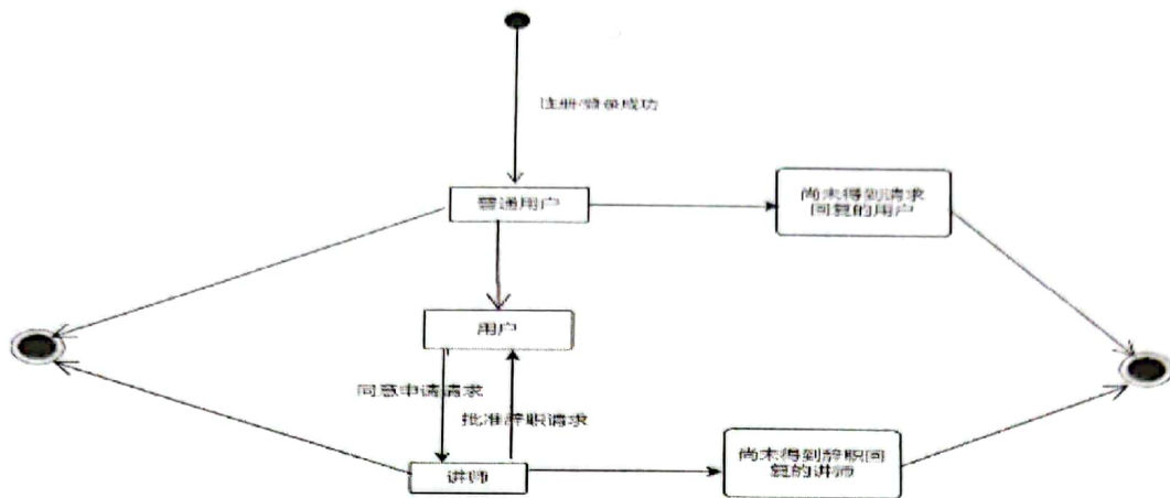
图 13 用户状态图
