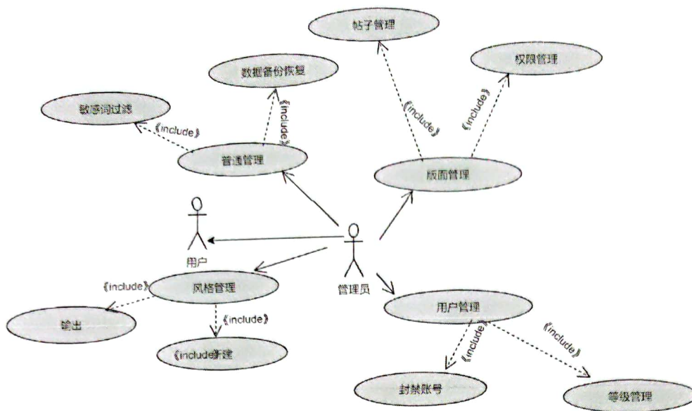
图 6 管理员用例图
