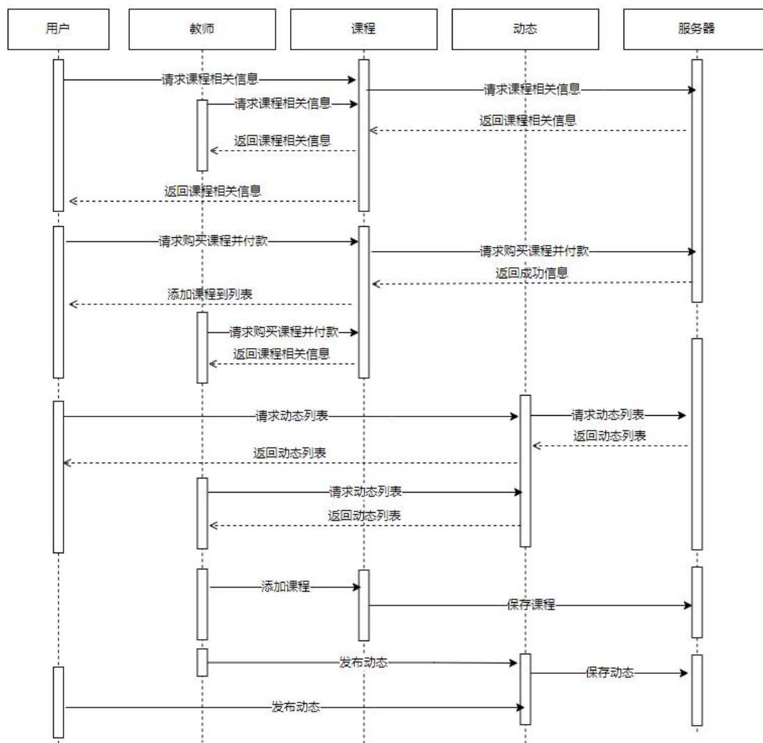
时序图二
