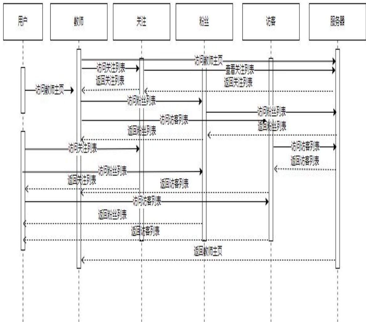
时序图一
