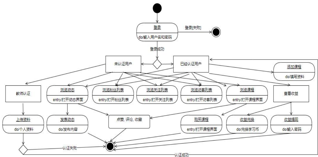
状态图
