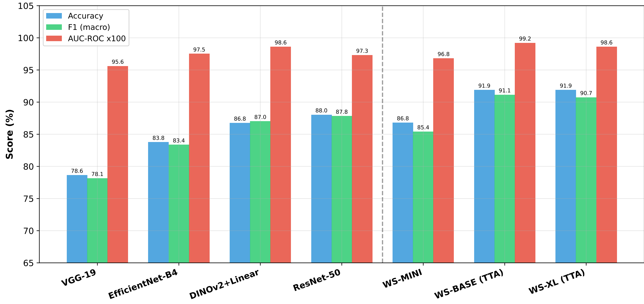
Classification Metrics: Accuracy / F1 / AUC-ROC
