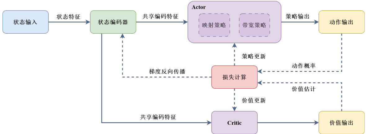
图 4-1 双分支策略网络架构
