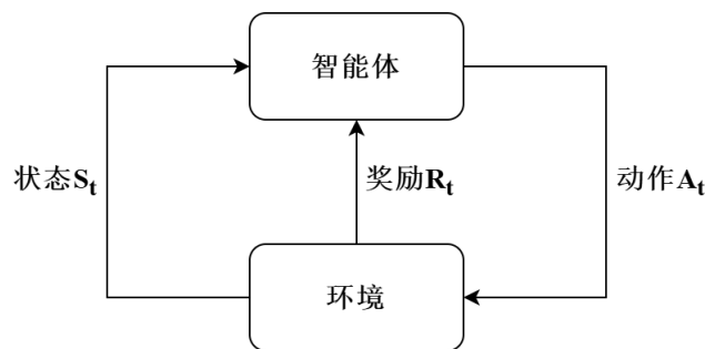
图 2-1 强化学习模型
