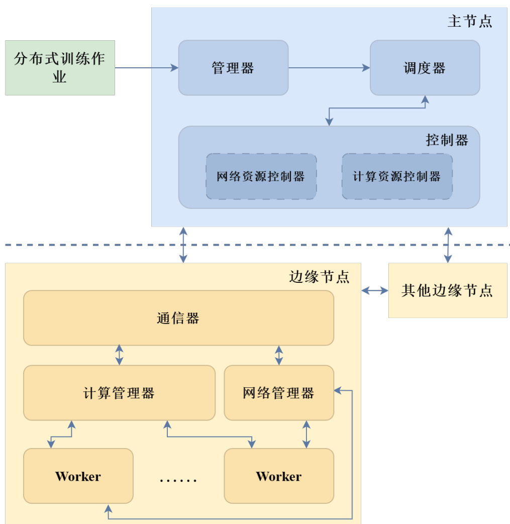
图 3-1 协同边缘任务调度系统 CES 架构图
