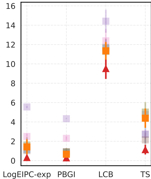
Volkert
