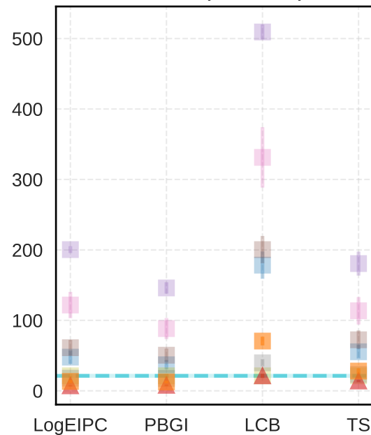
Dionis (416188)
