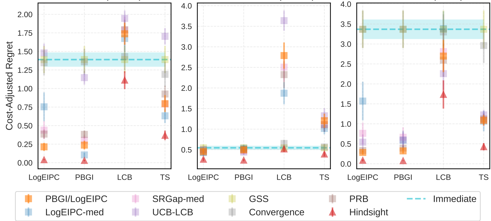
Nomao (34465)
