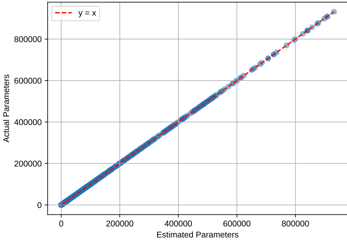
sylvine: Actual vs Estimated
