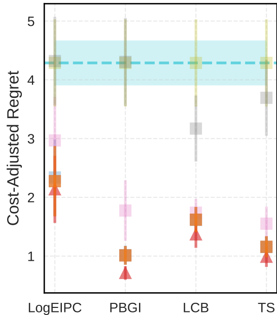
Kc1 (2109)
