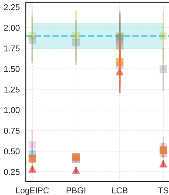
Kr-vs-kp (3196)
