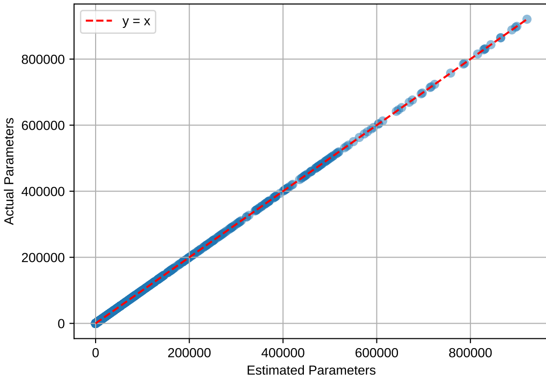
car: Actual vs Estimated
