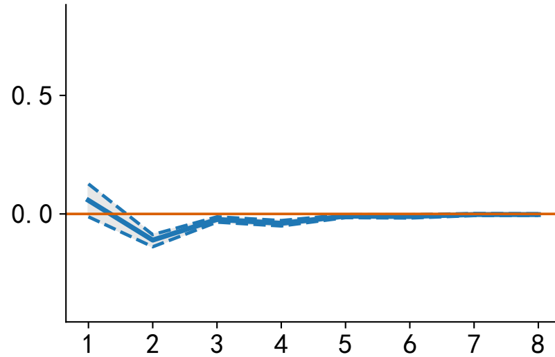
JP (CPI) → US (GDP)
