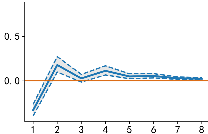
US (HUR) → US (GDP)
