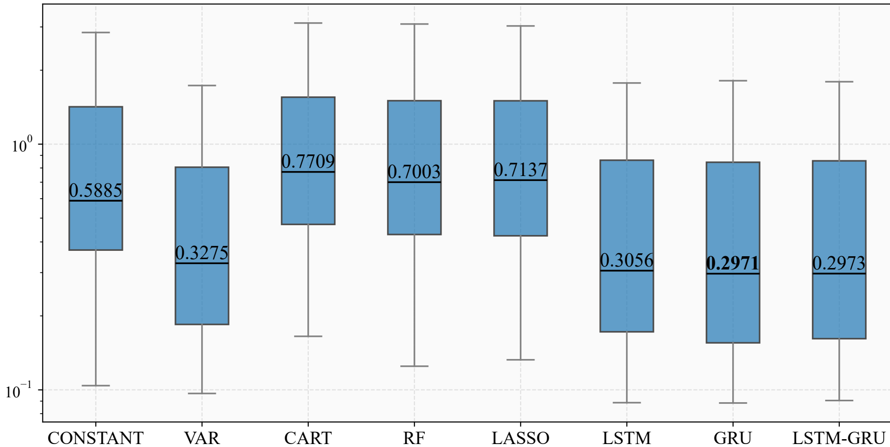
Macro-MSE
