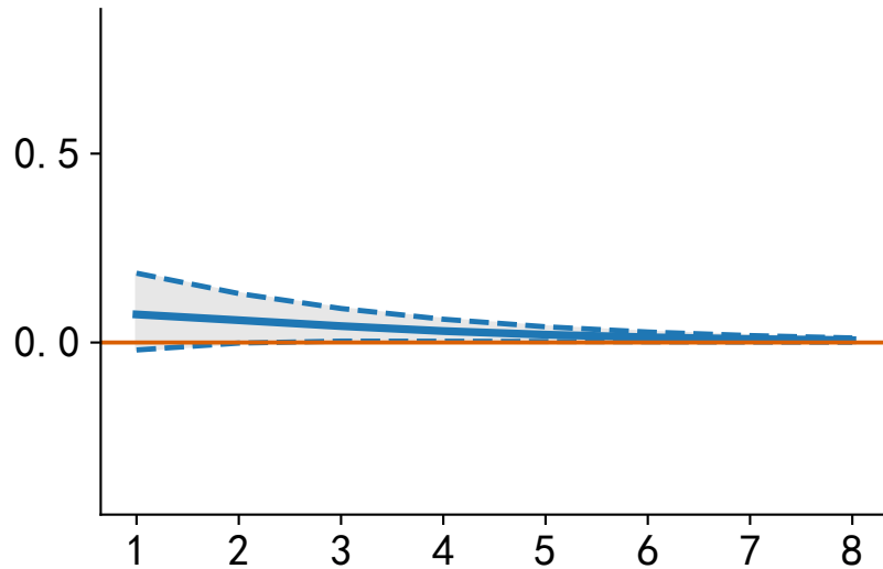
EU (CPI) → US (HUR)
