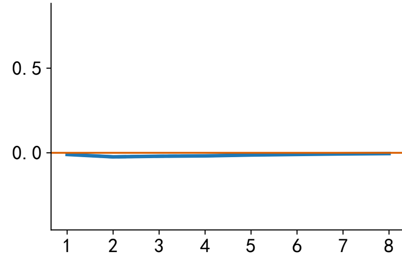
WTI → US (HUR)
