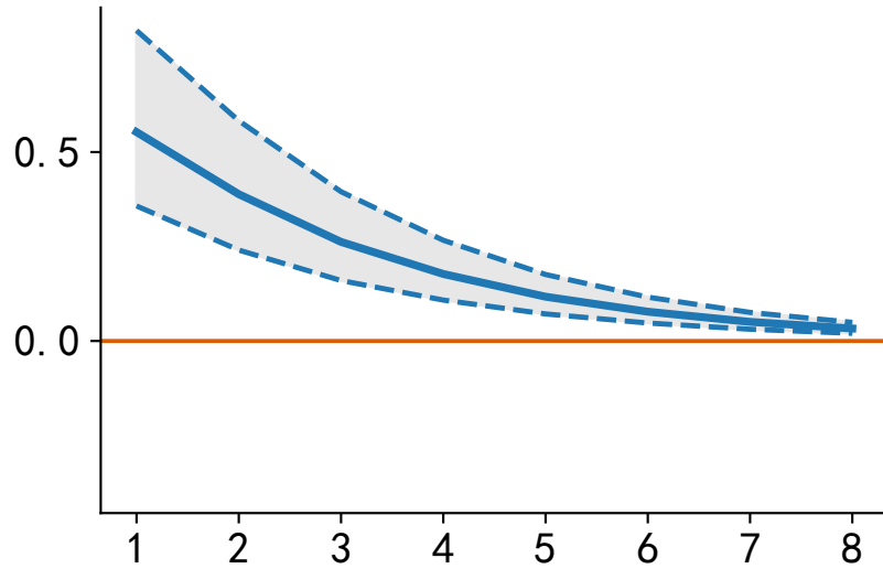
US (HUR) → US (HUR)
