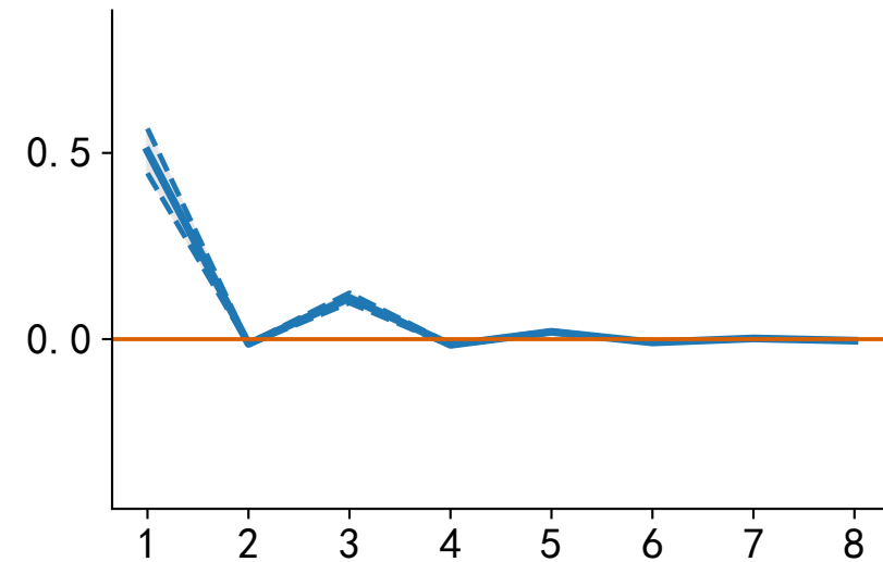
WTI → US (GDP)
