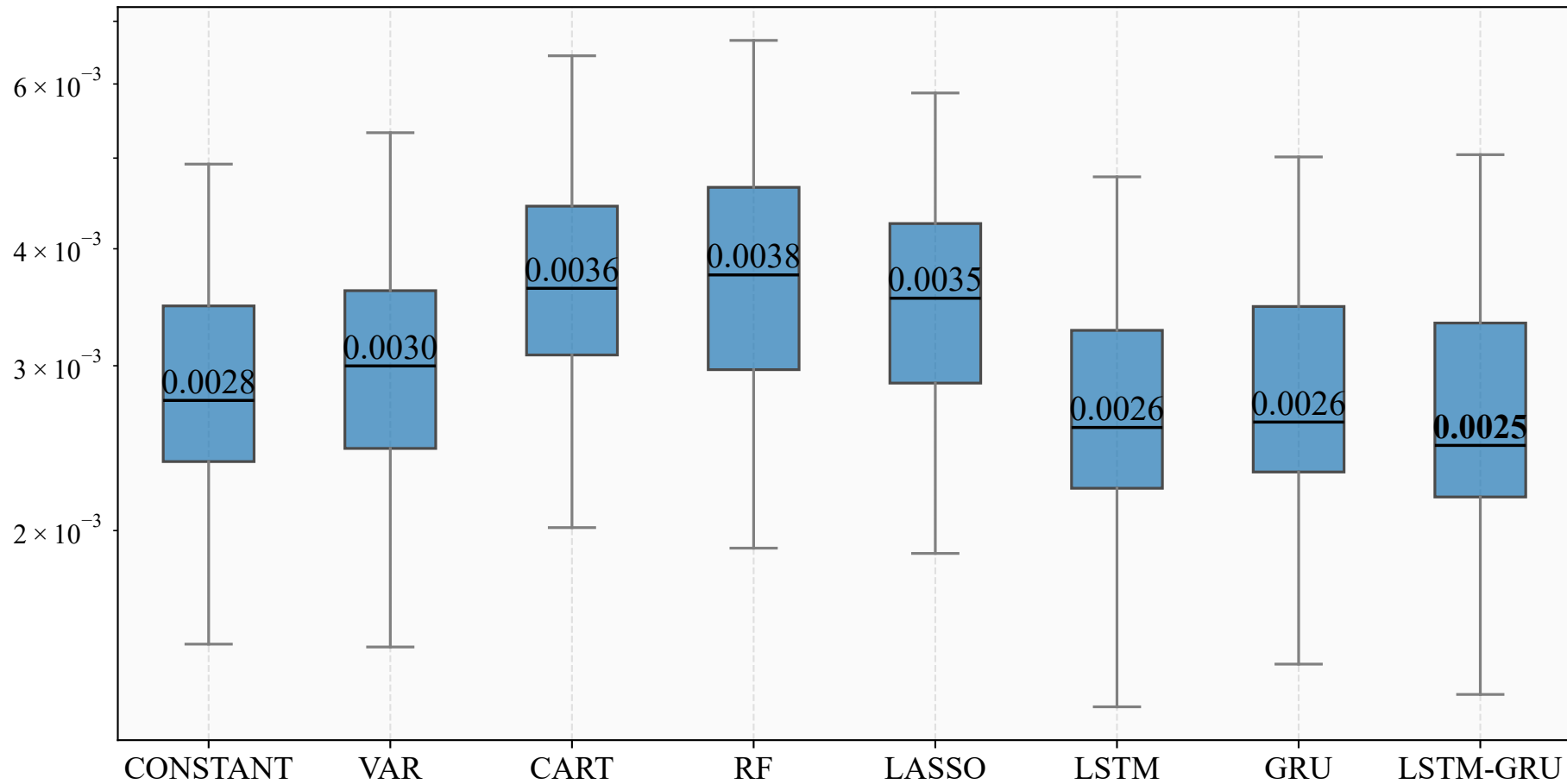
Macro-MSE
