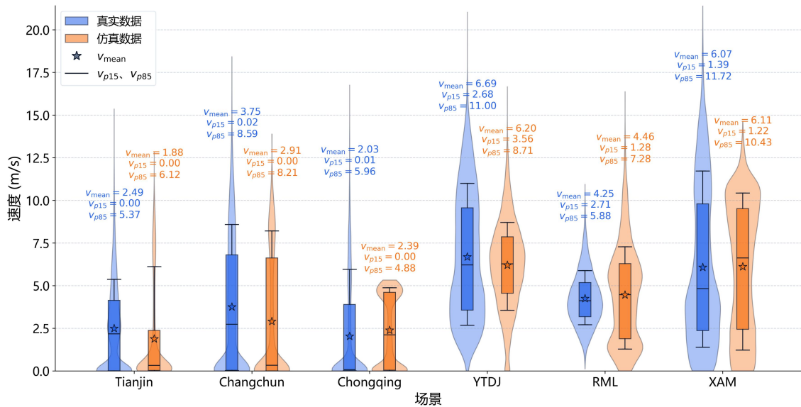
图 4.3 六场景标定前后速度分布对比小提琴图
