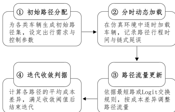
图 5 仿真方法求解流程
