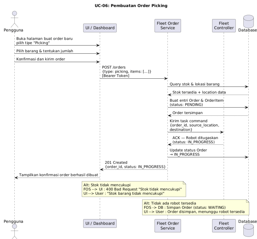
Gambar IV.20 Diagram sequence UC-06: Pembuatan Order Picking
