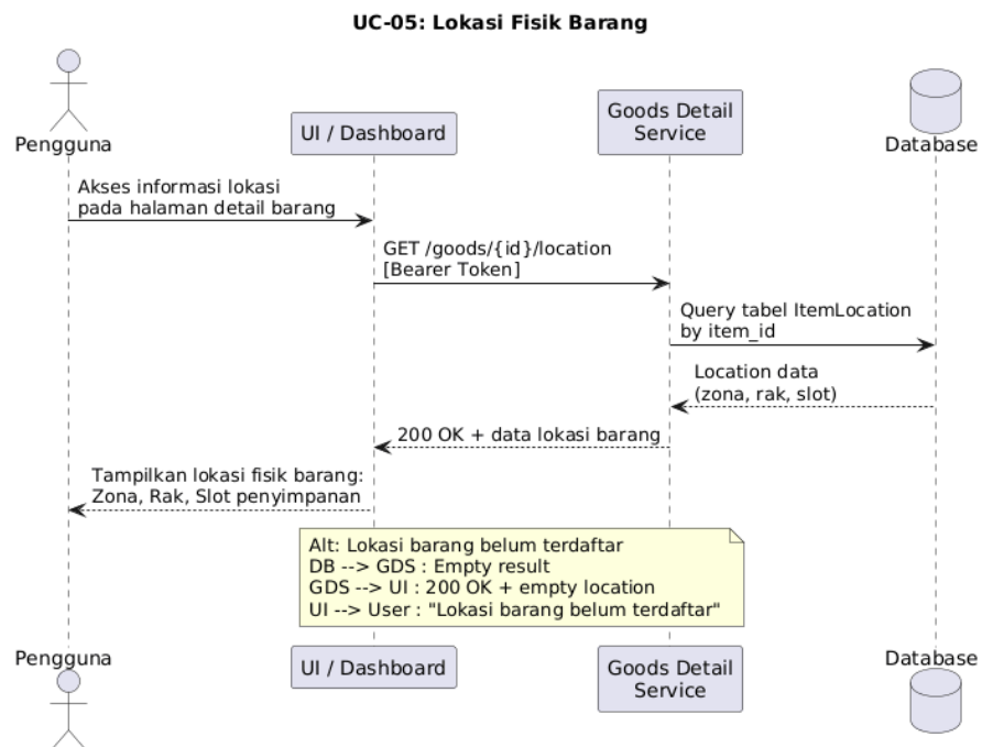
Gambar IV.19 Diagram sequence UC-05: Lokasi Fisik Barang
