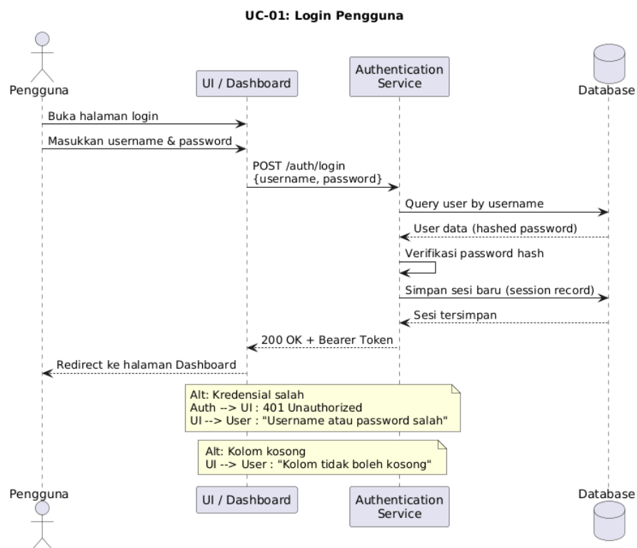
Gambar IV.15 Diagram sequence UC-01: Login Pengguna
