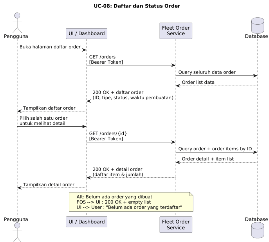
Gambar IV.22 Diagram sequence UC-08: Daftar dan Status Order
