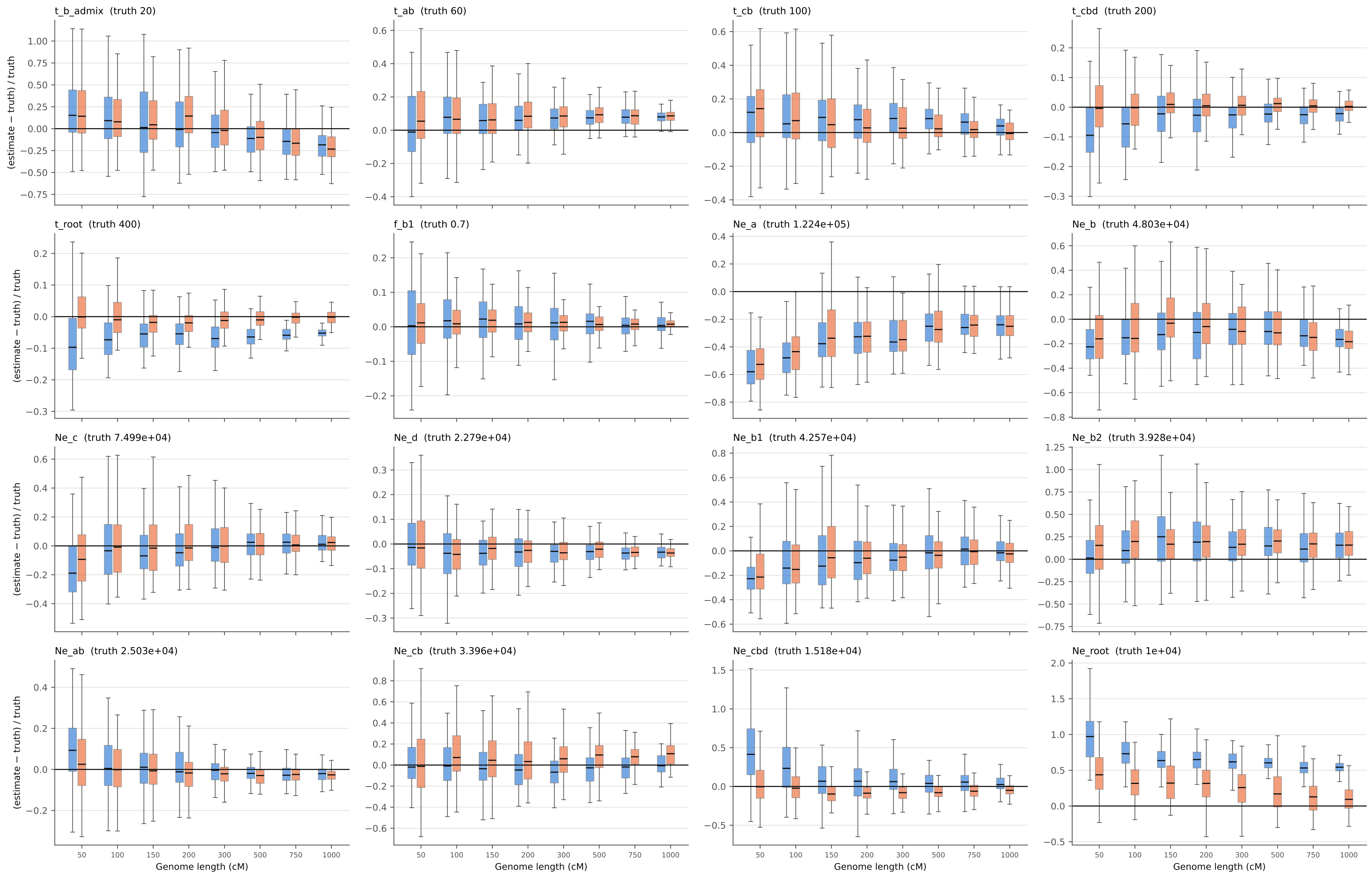
T_true parameter recovery: posterior means per subsample (Ne haploid)
