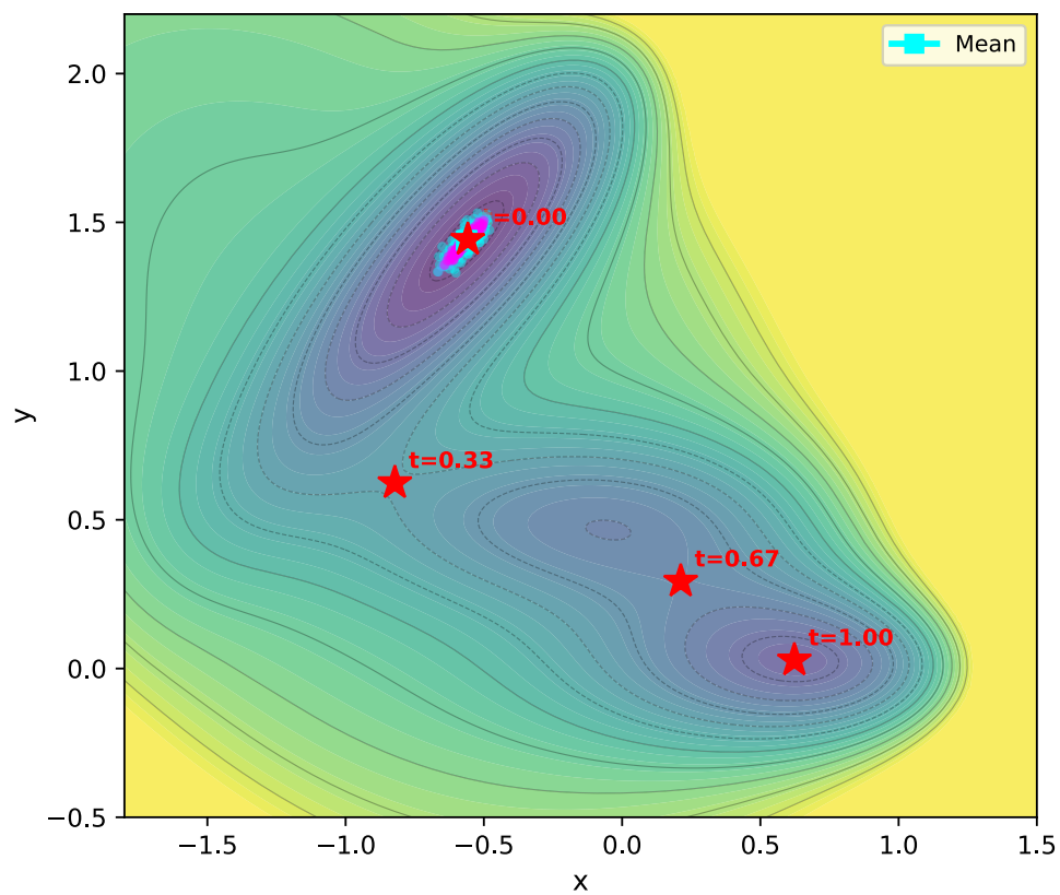
Algorithm 3 (JKO / Wasserstein)
