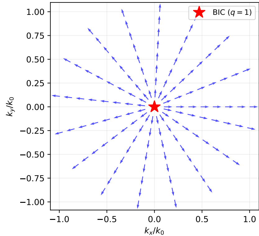
(a) Polarisation vortex ( q = 1 )
