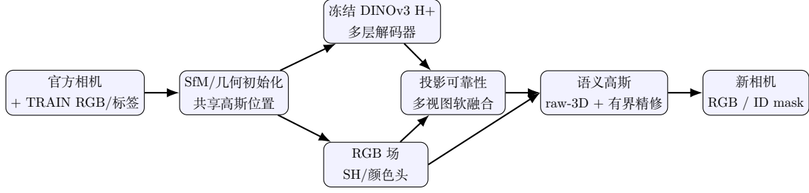
图 1: 训练与推理数据流：语义场内部共享 RGB 与语义几何，最终 RGB 来自两个独立 RGB 场；教师支路表示部署阶段前向。测试相机不需要真实目标照片，但仍需 DINOv3 H+ 及解码器。
