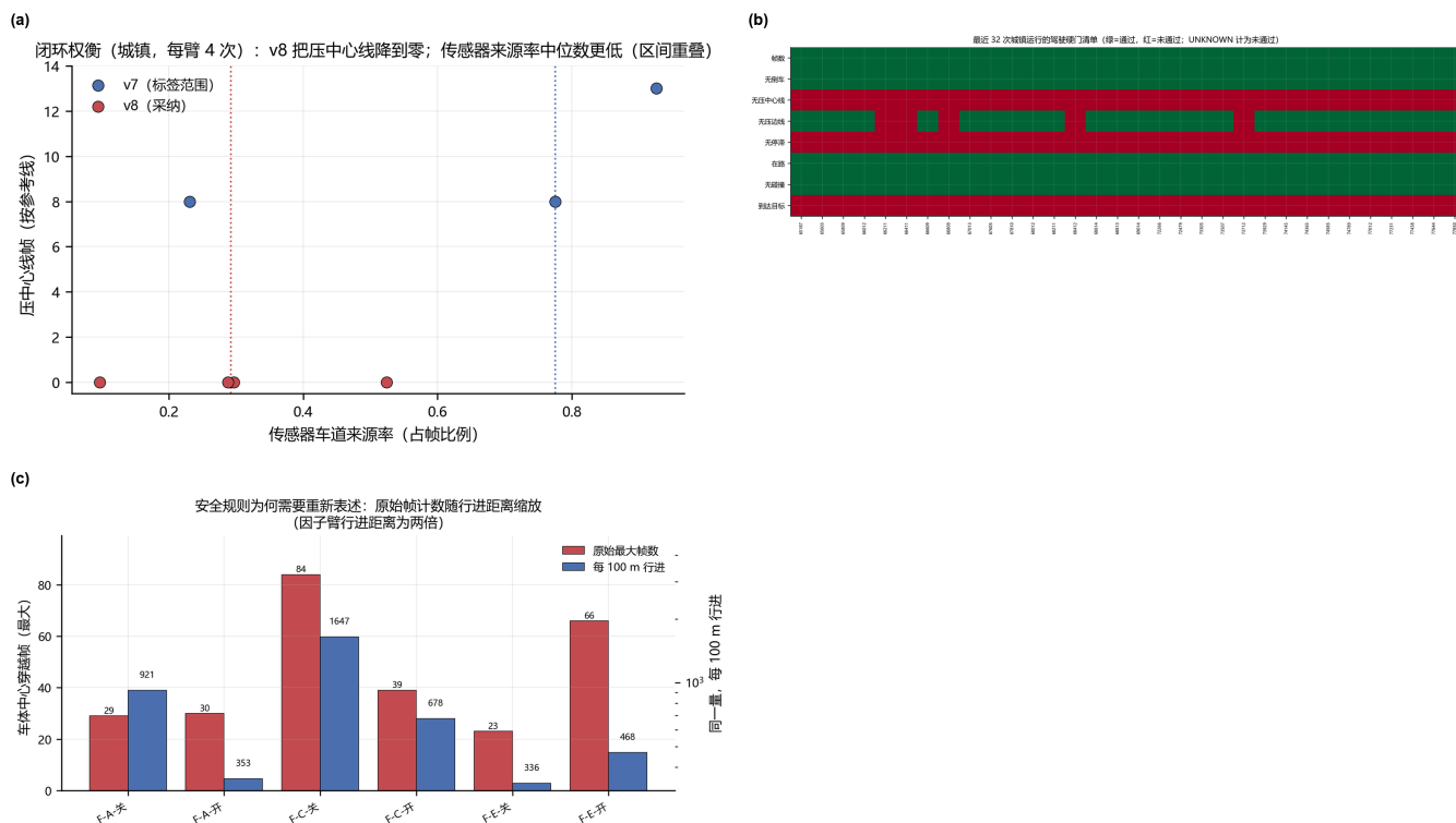
图 7. 闭环: (a) 两套定义下的压中心线与传感器车道来源率, (b) 最近各次城镇运行的硬目标清单, (c) 安全规则为何需要重新表述 (原始计数随行进距离缩放)。
