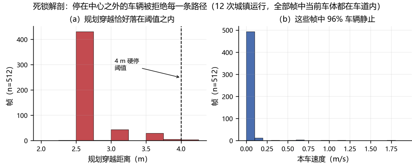
图 7. 死锁解剖：规划穿越恰好落在 4 m 阈值之内 (a)，且在这些帧中车辆 96% 时间静止 (b)。
