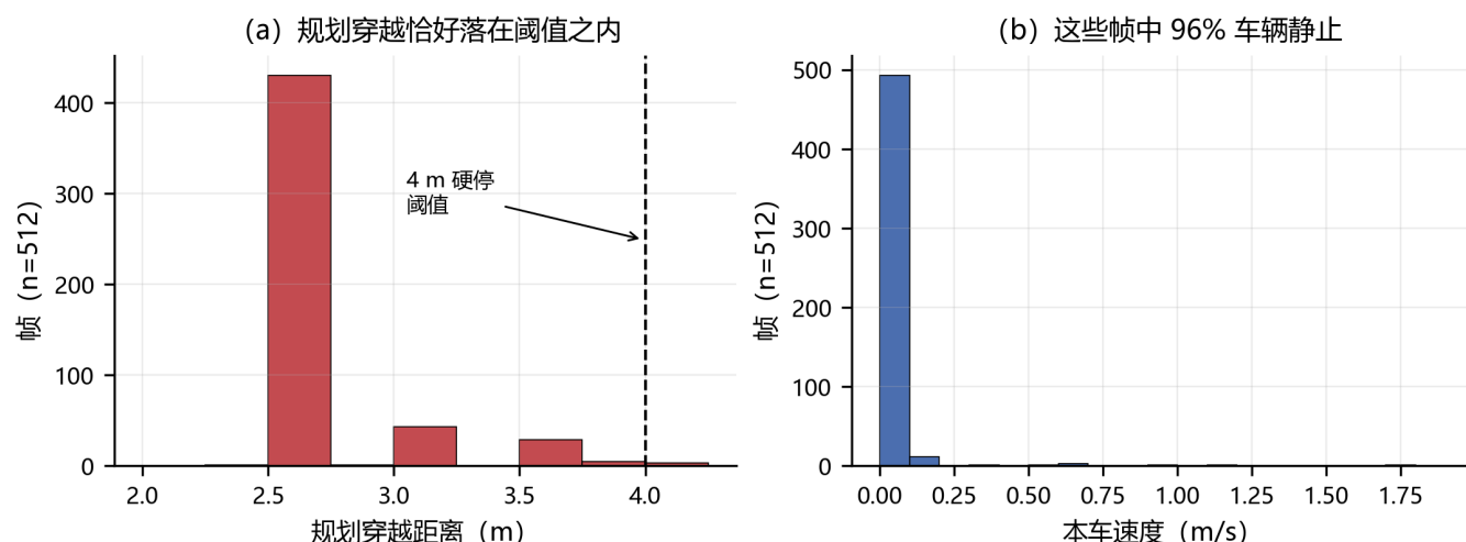
图 7. 死锁解剖：规划穿越恰好落在 4 m 阈值之内 (a)，且在这些帧中车辆 96% 时间静止 (b)。
