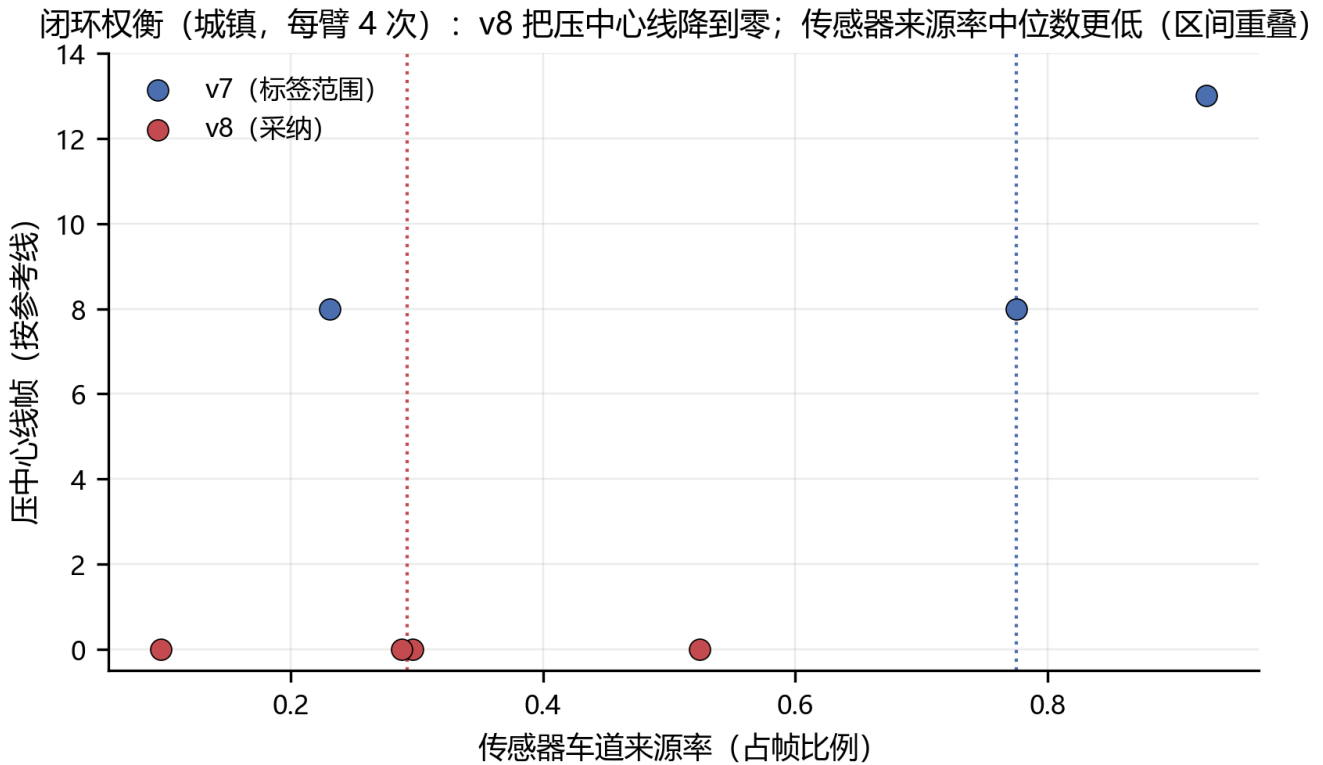
图 6. 闭环权衡：中心线穿越与传感器车道来源率，每臂四次运行。
