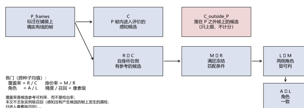
图 3. 计数契约（示意）：每个比率都在冻结的计数定义上有显式分子与分母；覆盖率是候选参考可判率，不是检出率。
