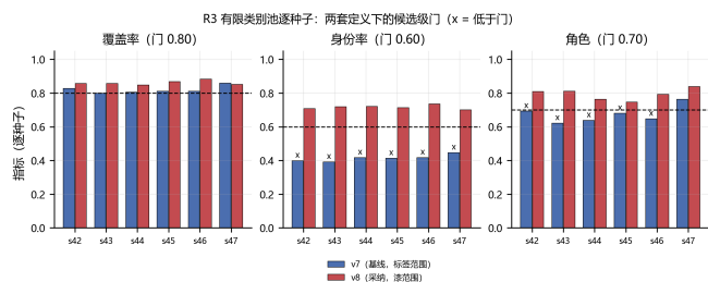
图 10. 有限类别池逐种子：两套定义下的三个候选级门，与表 I 取自同一批判定文件（x = 低于门）。
