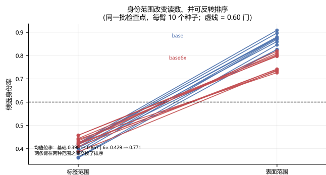
图 12. 身份范围改变读数、并可反转排序：20 个检查点（两条臂、每臂 10 个种子）在标签范围与表面范围下的读法。
