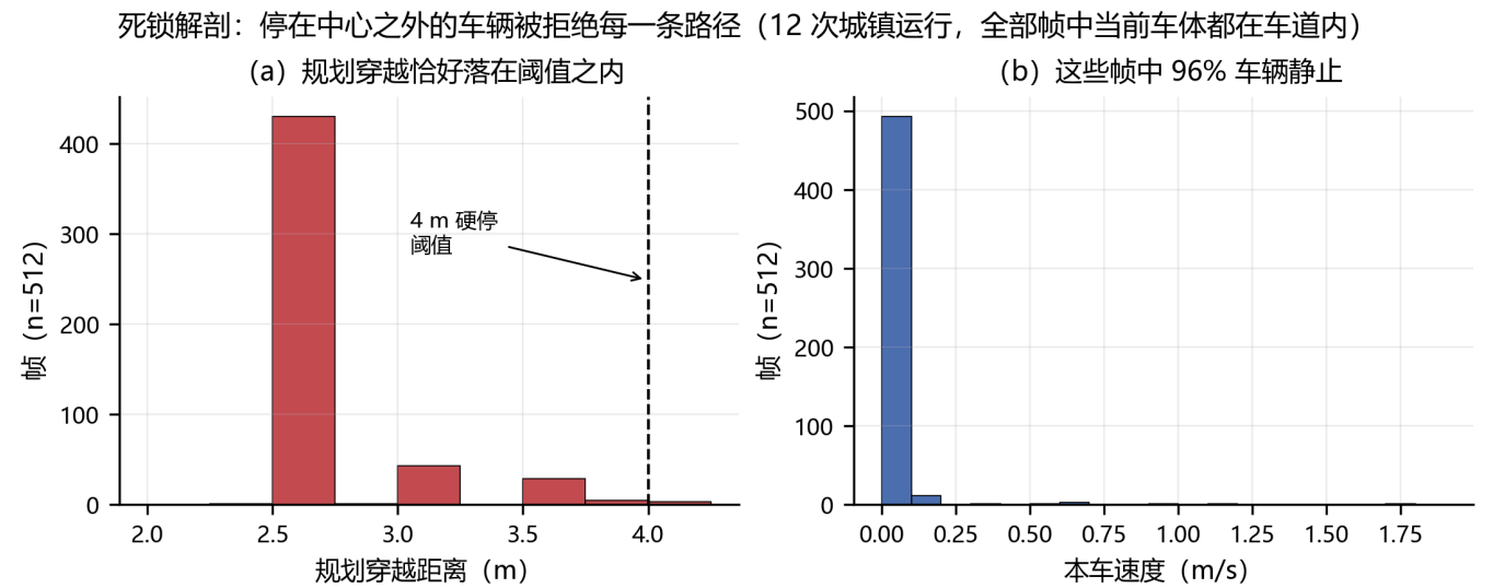
图 7. 死锁解剖：规划穿越恰好落在 4 m 阈值之内 (a)，且在这些帧中车辆 96% 时间静止 (b)。
