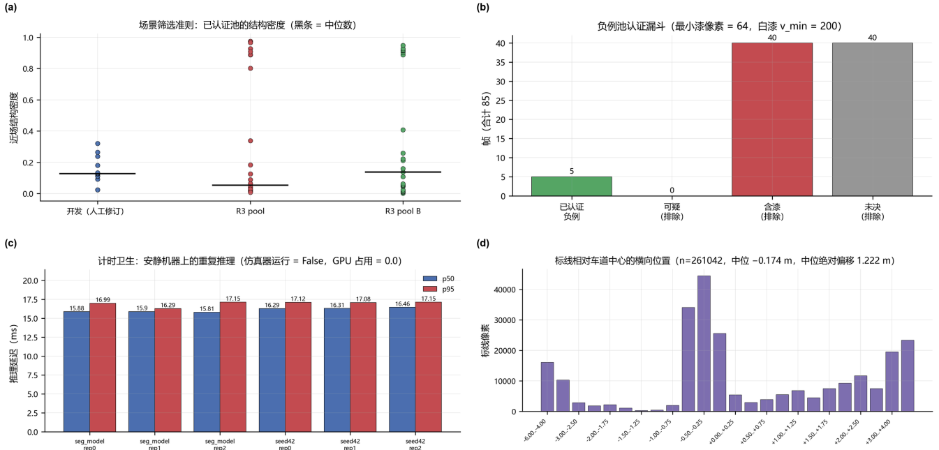
图 3. 严谨性与审计：(a) 场景筛选准则（近场结构密度），(b) 负例池认证漏斗，(c) 计时卫生复测，(d) 参考标线的实测横向几何。
