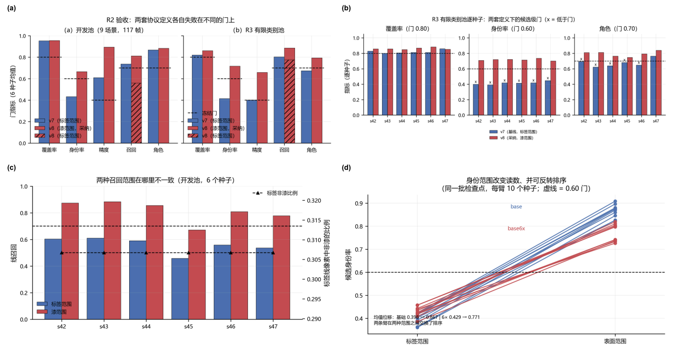
图 4. 验收结果的定义敏感性: (a) 两套协议定义下的门指标与冻结阈值, (b) 两套定义下有限类别池逐种子 ( x = \text{低于门} ), (c) 标签范围与漆范围召回并叠加标签线像素的非漆比例, (d) 同一批检查点在标签范围与表面范围身份下的读法——两条臂在这里交换了排序。
