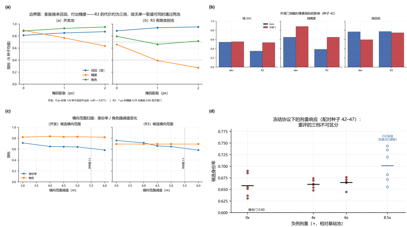
图 5. 后处理与组成的单因子：(a) 边界图（掩码膨胀），(b) 外观门对像素指标的消融，(c) 横向范围扫描，(d) 候选身份率随负例剂量的响应。
