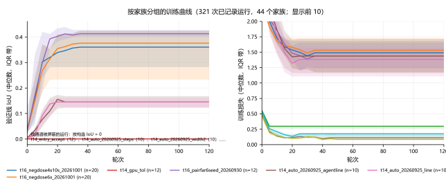
图 S14. 已记录 `train_hist.json` 运行的训练曲线（逐轮次验证线 IoU 与训练损失）。
