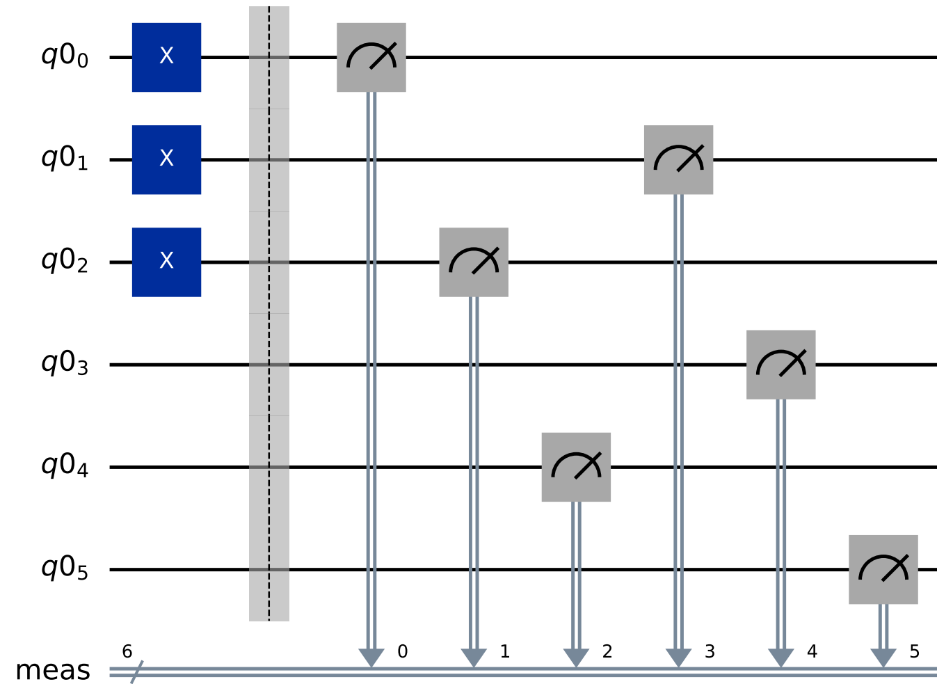
transpiled
