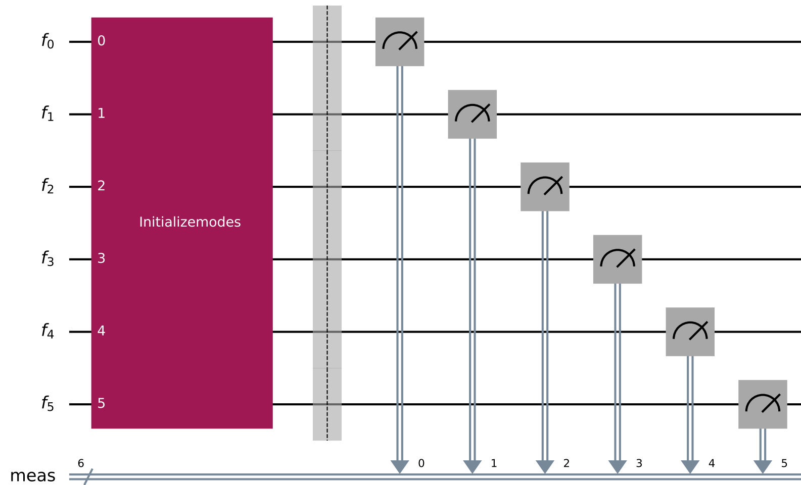
fermionic
